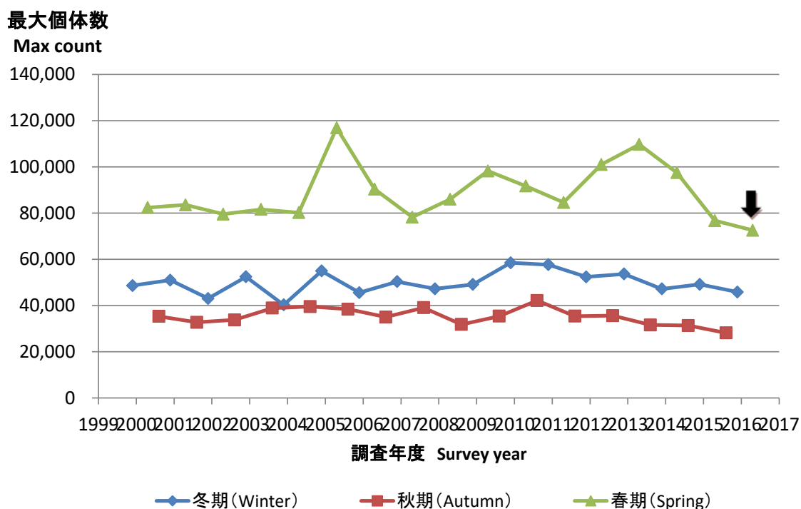
図 7. 全サイトにおけるシギ・チドリ類の最大個体数の動態
