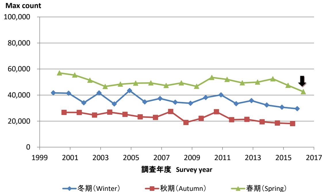
図 8-3. 1999 年以降連続して調査が行われたサイトにおけるヒレアシシギ類を除いた最大個体数の動態 継続サイトは春期調査で 45 サイト、秋期調査 52 サイト、冬期調査 44 サイト。
