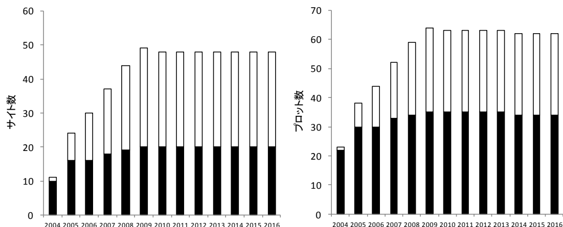
図Ⅱ-3-1. 2004-2016 年度のコアサイト・準コアサイト数及び調査区数の推移
