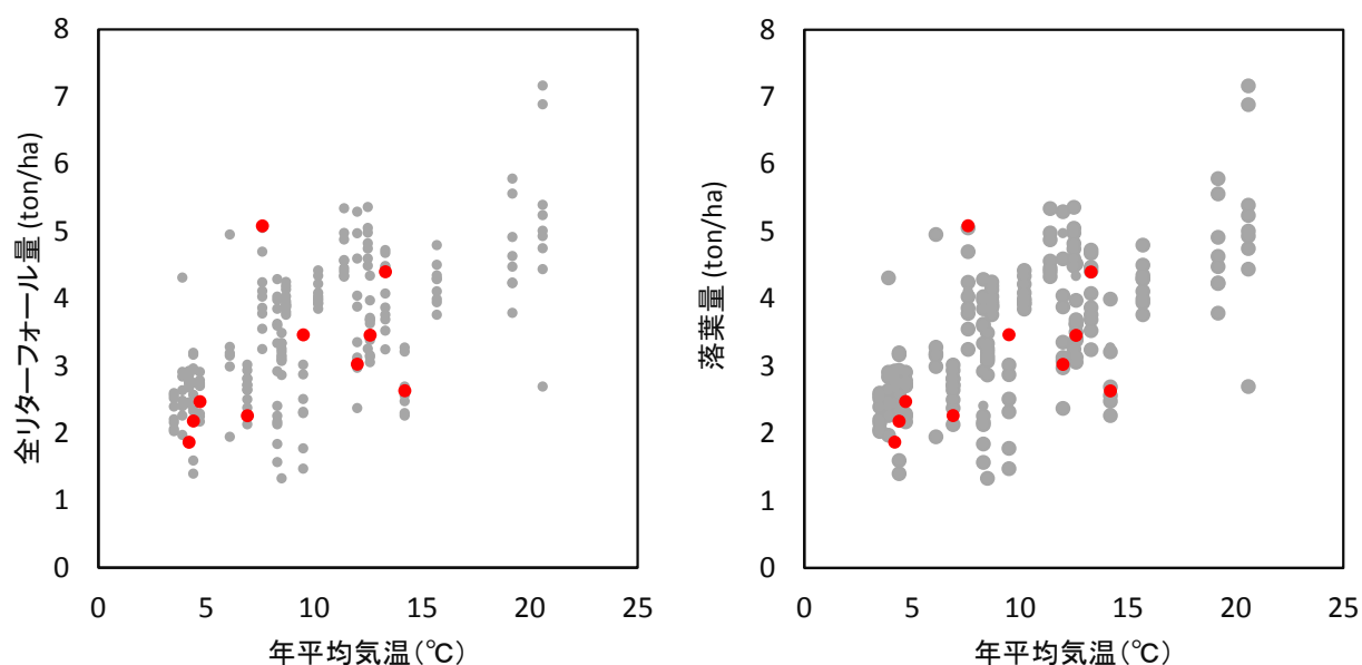
図Ⅱ-1-1. 2004～2014年度(灰色)及び2015年度(赤色)の年間落葉量及びリターフォール量と年平均気温の関係。
