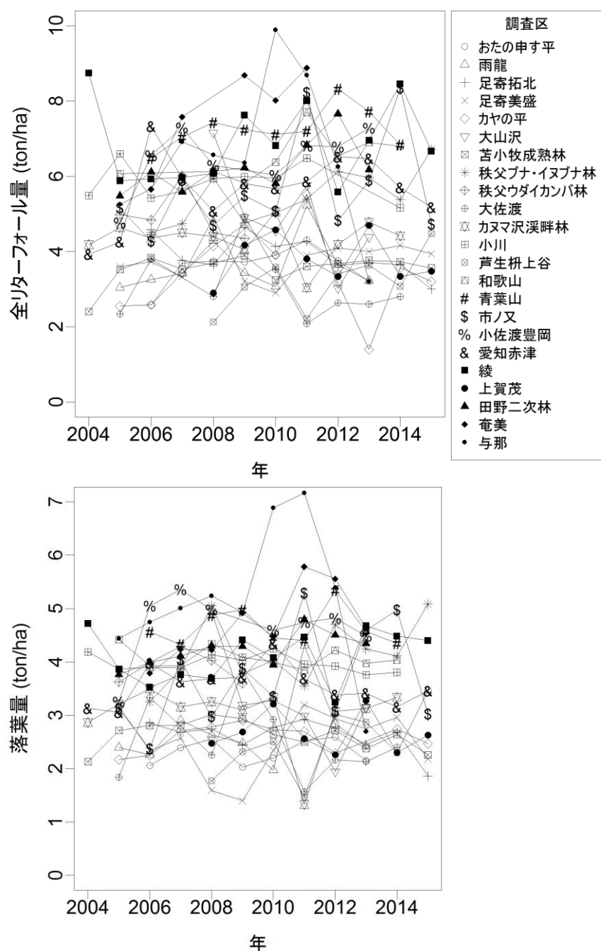
図Ⅱ-1-2. 年間リターフォール量(上)と年間落葉量(下)の年変動。
