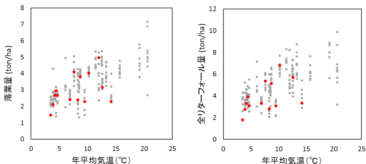
図Ⅱ-1-1. 2004～2014年度(灰色)および2015年度(赤色)の年間落葉量およびリターフォール量と年平均気温の関係。
