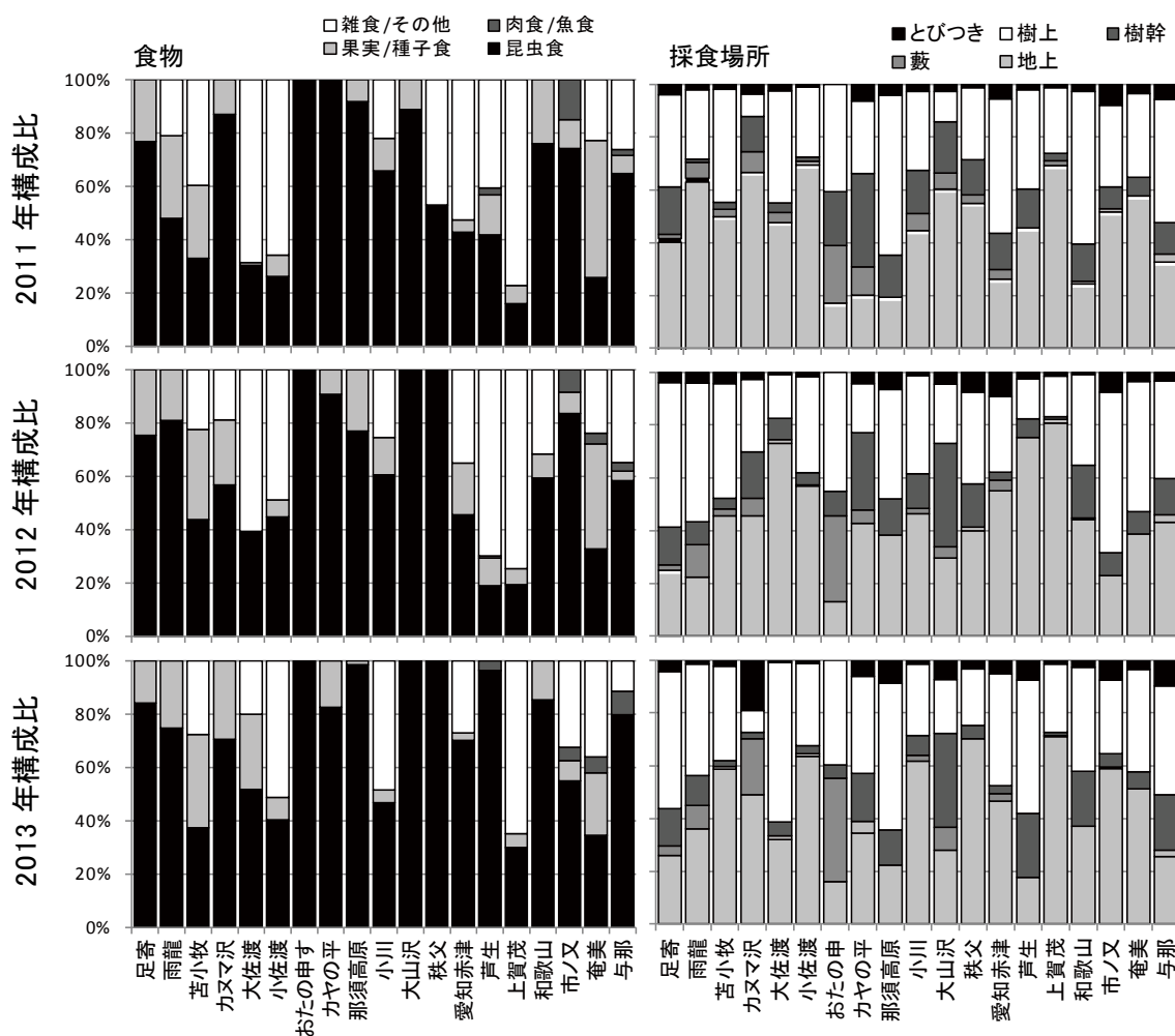
図Ⅱ-5-3. 2011-2013 年度繁殖期に記録された食物別、採食場所別の鳥類のバイオマスの割合 左ほど寒冷な調査地
