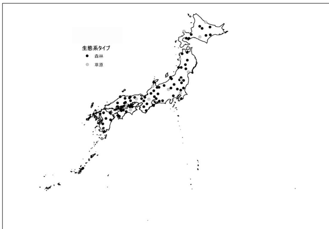
図Ⅲ-1-1. 2013年度調査依頼サイト
