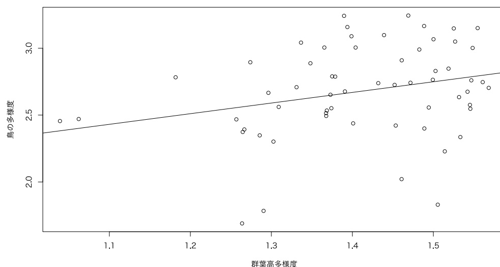
図Ⅲ-3-1. 森林サイトの群葉高多様度と鳥類の種多様度の関係
