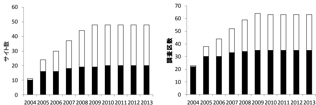
図Ⅱ-1-1. 2004-2012 年度のコアサイト・準コアサイト数及び調査区数の推移
