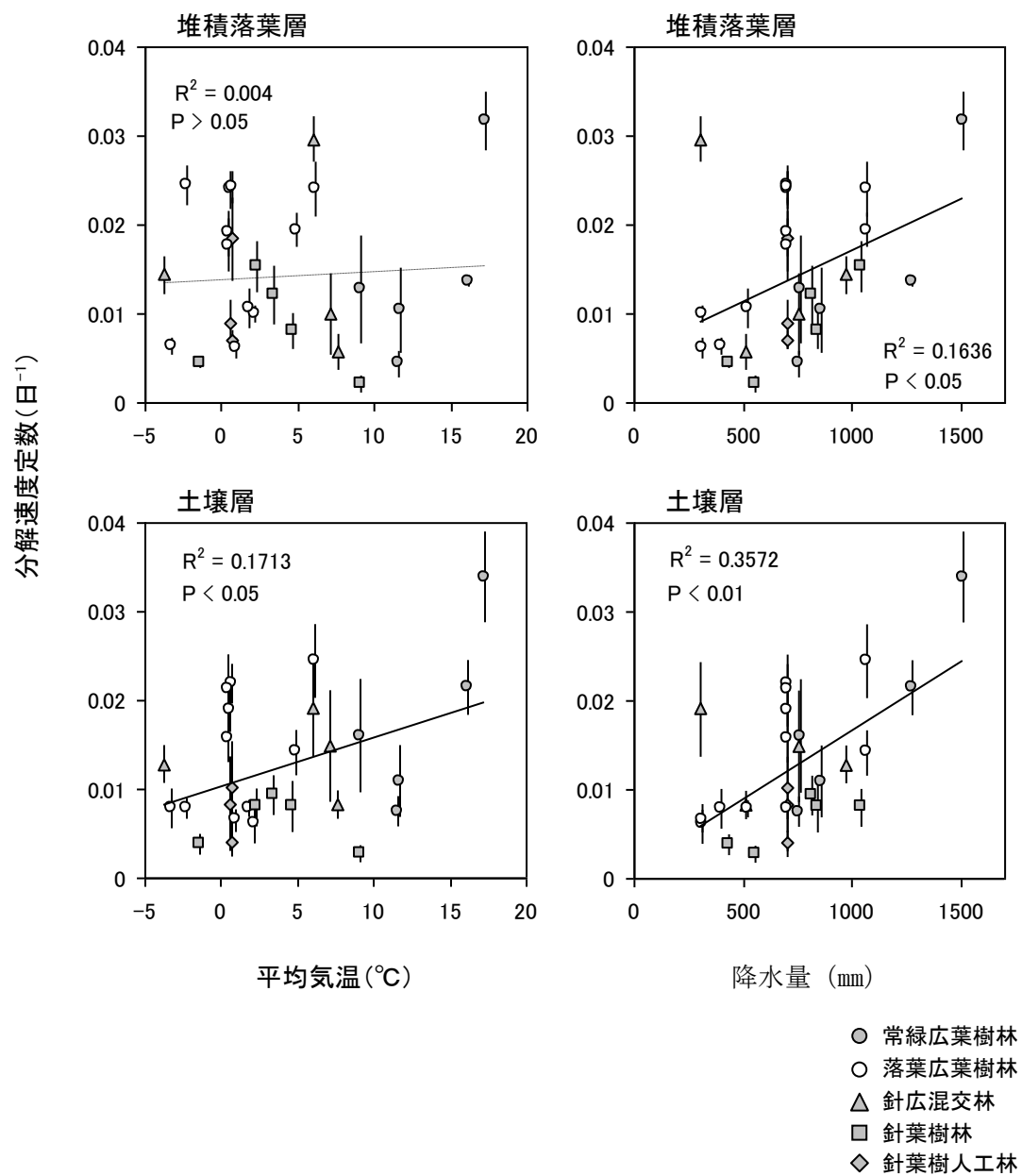
図 II-4-3. セルロース紙の分解速度定数(5サブプロットの平均±標準誤差)と設置期間中の気象条件(2012年11月～2013年5月)との関係
