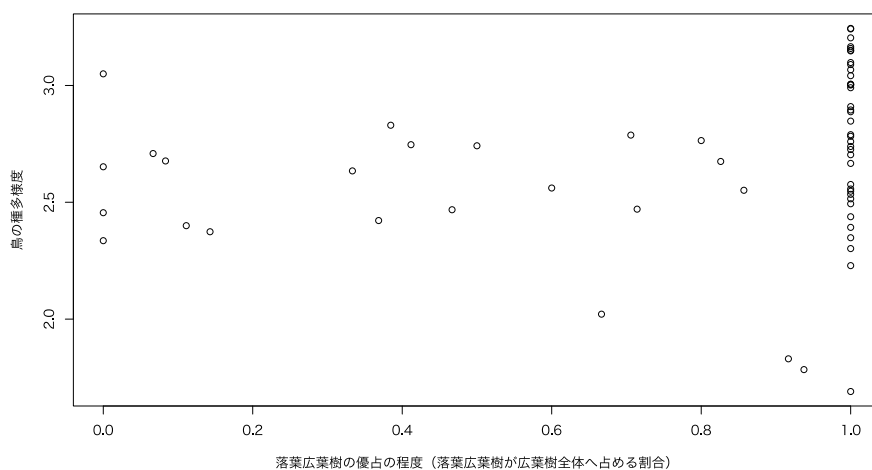
図 III-3-2a. 森林サイトの群葉高多様度と鳥類の種多様度の関係
