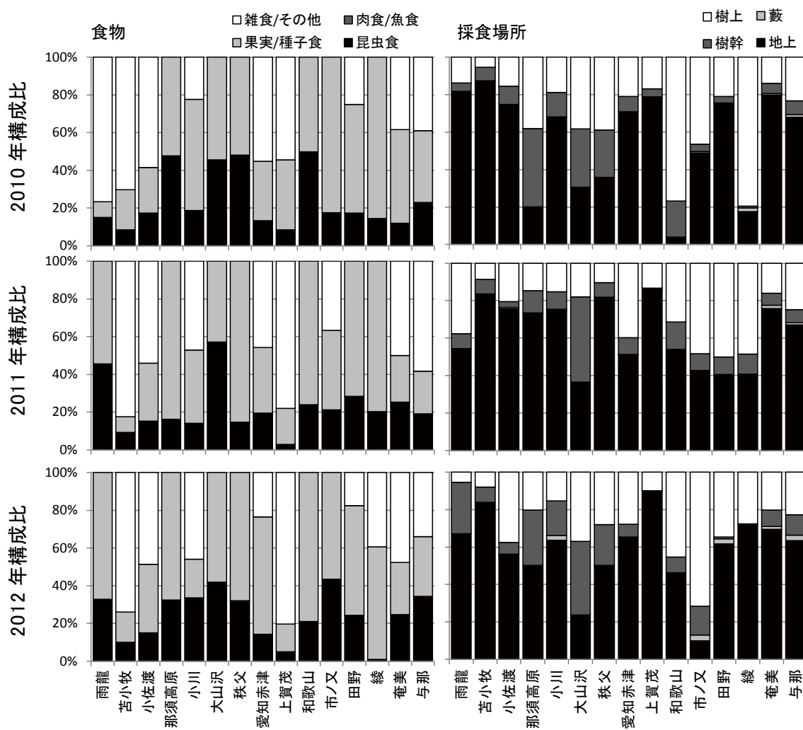
図 II-5-2. 2010～2012 年度越冬期に記録された食物別、採食場所別の鳥類のバイオマスの割合
