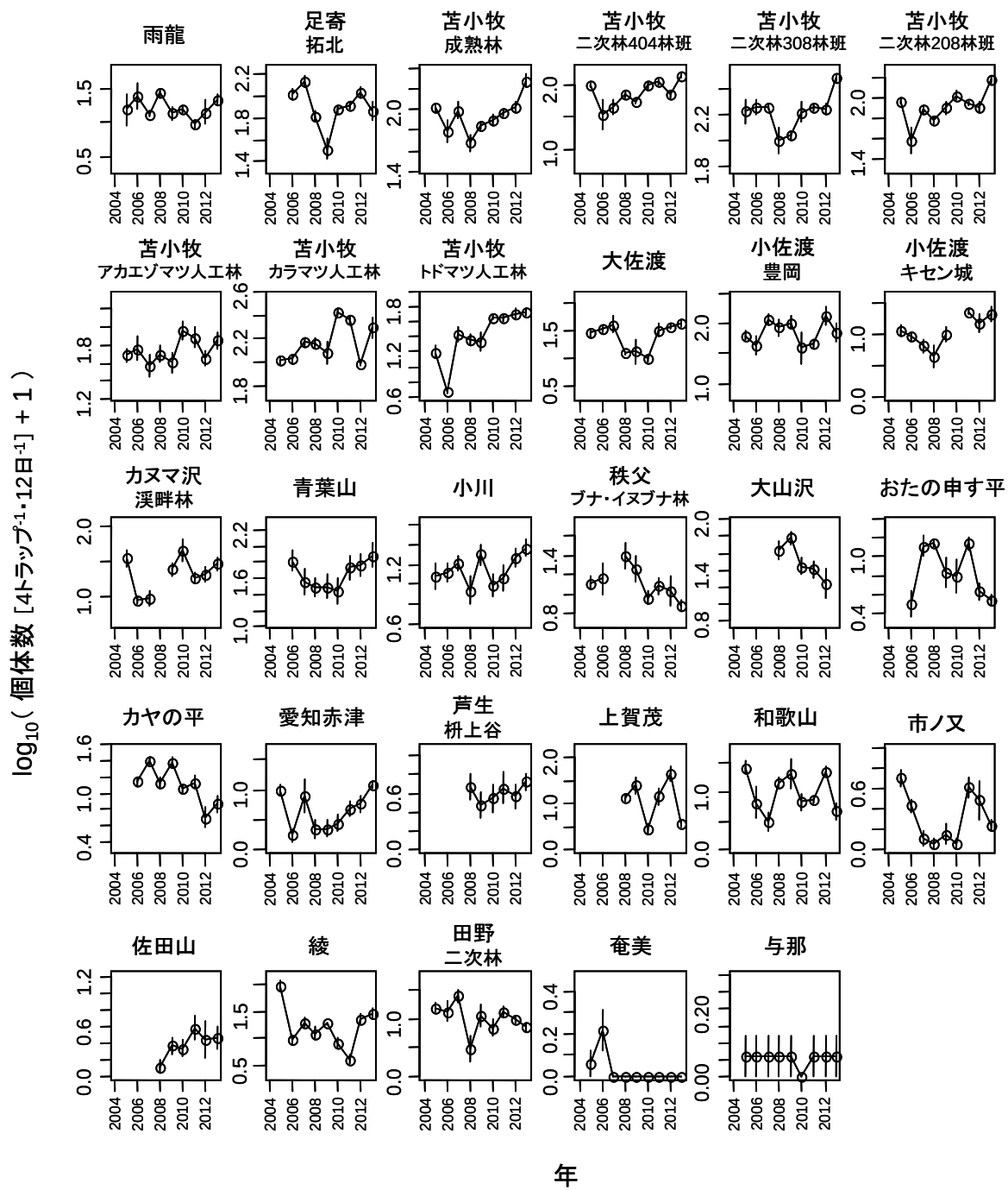
図 II-4-1. 各調査区における地表徘徊性甲虫類の捕獲個体数の年変動(5サブプロットの平均±標準誤差)
