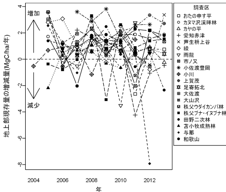
図Ⅱ-2-2. 2004～2013 年度のコアサイトにおける地上部現存量の増減量の推移
