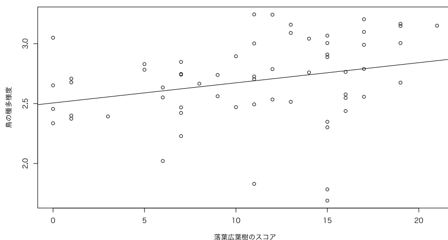
図 III-3-2b. 森林サイトの落葉広葉樹のスコアと鳥類の種多様度の関係
