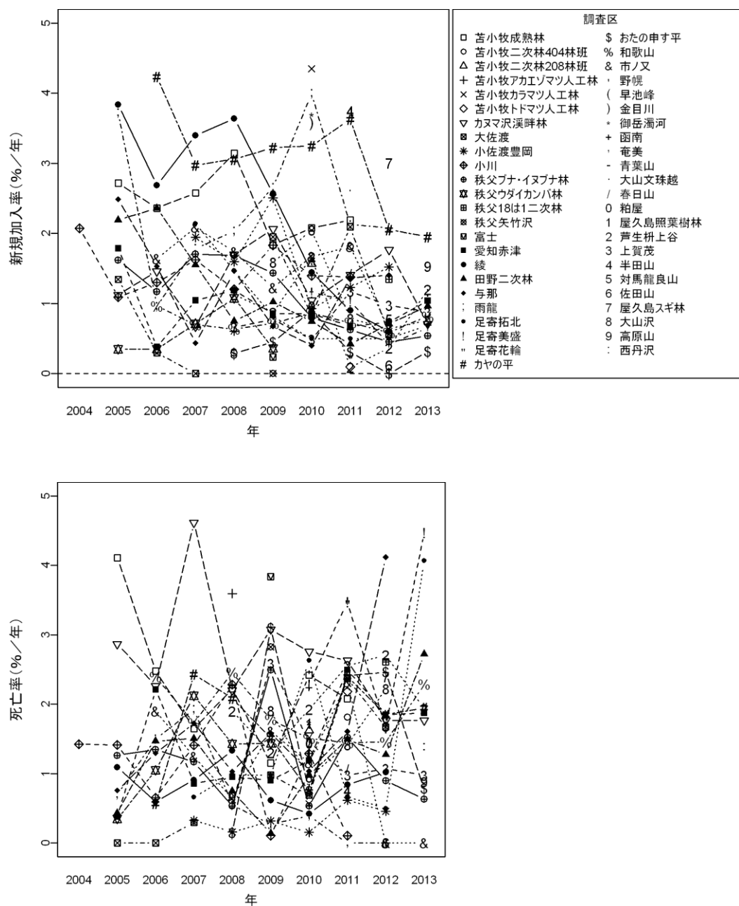
図 II-2-4. 2004～2013 年度の新規加入率、死亡率、回転率の変化
