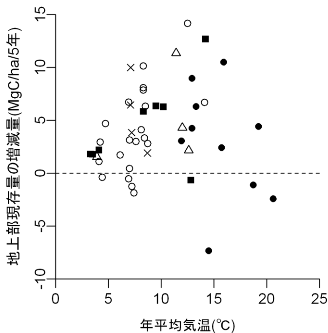
図Ⅱ-2-3. 調査開始時からの地上部現存量の増減量と年平均気温の関係 増減量は5年あたりに換算した値。常緑針葉樹林 ■、針広混交林 △、落葉広葉樹林 ○、常緑広葉樹林 ●、×人工林。
