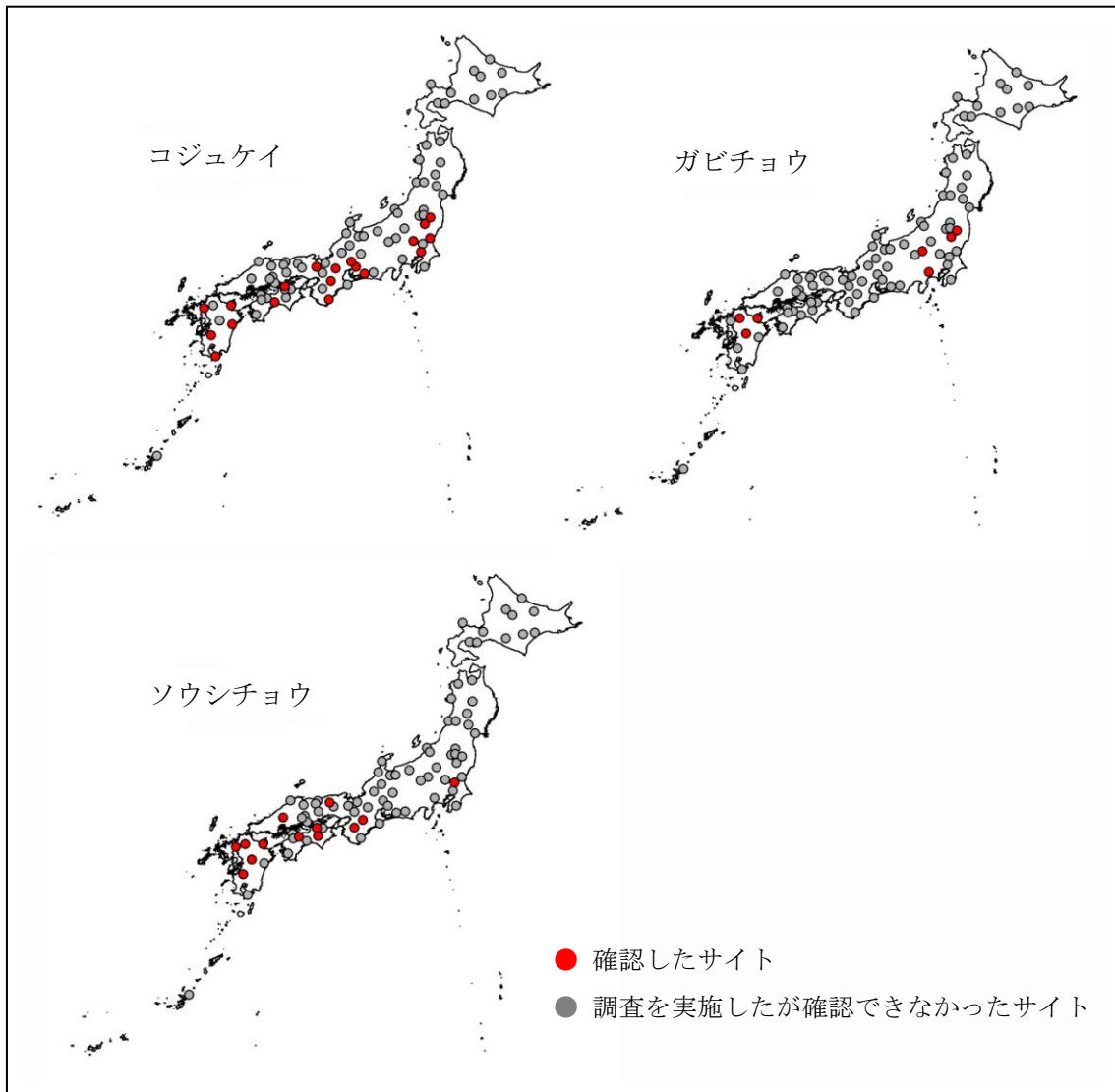
図 III-3-4. 2013 年度繁殖期における外来種 3 種の記録地点体数
