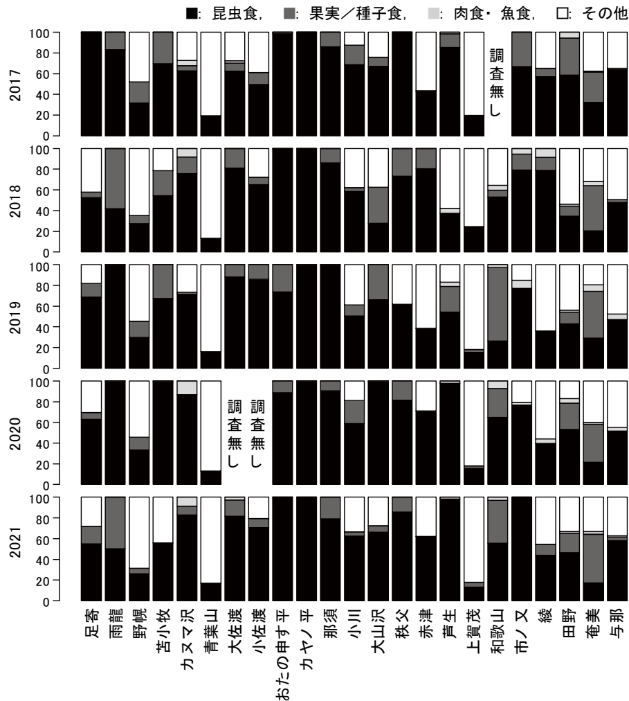
図Ⅱ-5-4. 2017-2021 年度繁殖期に記録された鳥類の食性別のバイオマス割合
