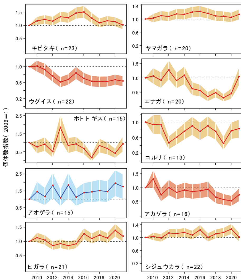
図Ⅱ-5-6. 2009年以降の各種鳥類の繁殖期の記録数の変遷
