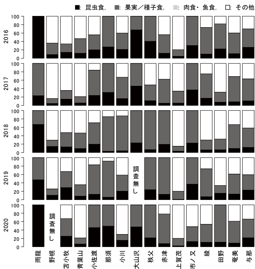
図Ⅱ-5-1. 2016-2020 年度越冬期に記録された鳥類の食性別のバイオマス割合
