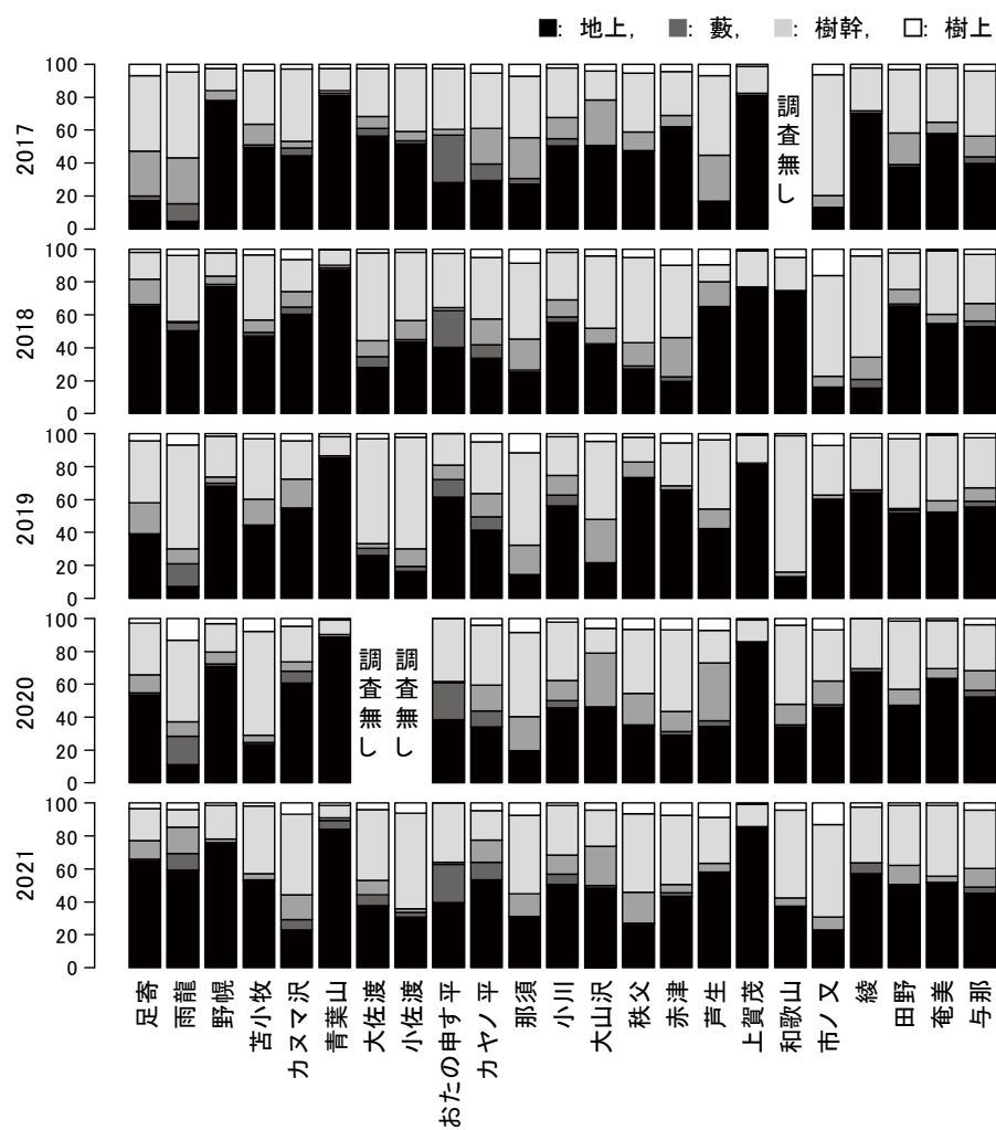
図Ⅱ-5-5. 2017-2021 年度繁殖期に記録された採食場所別のバイオマス割合
