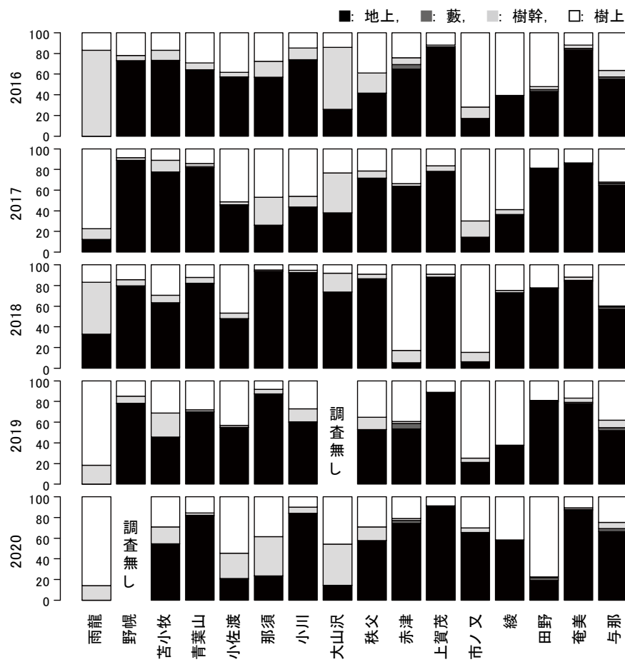
図Ⅱ-5-2. 2016-2020 年度越冬期に記録された鳥類の採食場所別のバイオマス割合
