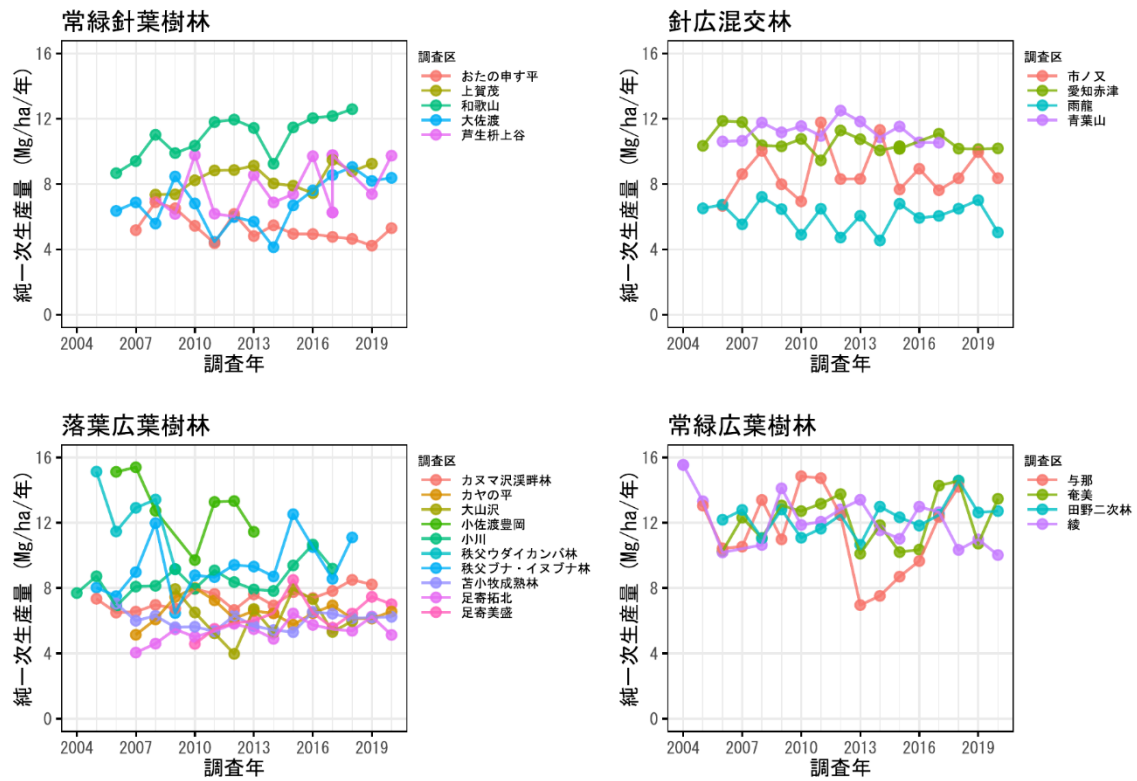
図Ⅱ-3-3. 各調査区における年間純一次生産量の時系列変化
