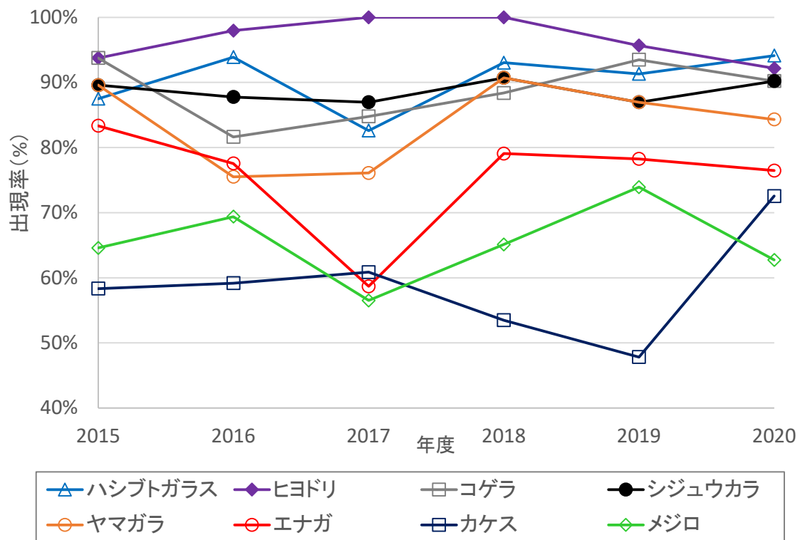
図Ⅲ-2-2. 出現率上位種における過去6年間（最新年度+過去5年）の推移（森林・越冬期）
