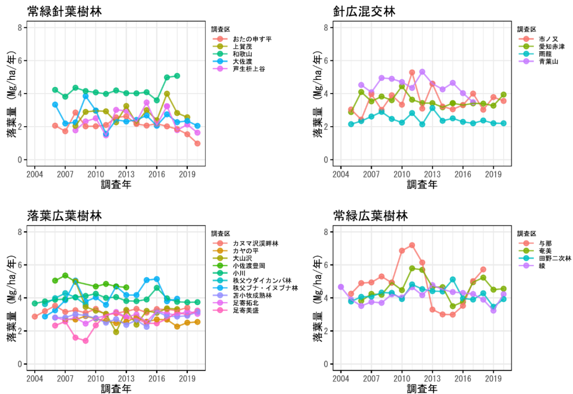
図Ⅱ-3-2. 各調査区における年間落葉量の時系列変化
