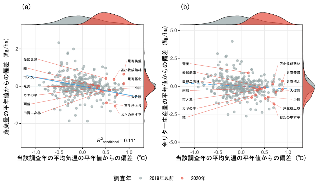
図Ⅱ-3-4. 年間落葉生産量(a)及び全リター量(b)の変動と気温変動の関係
