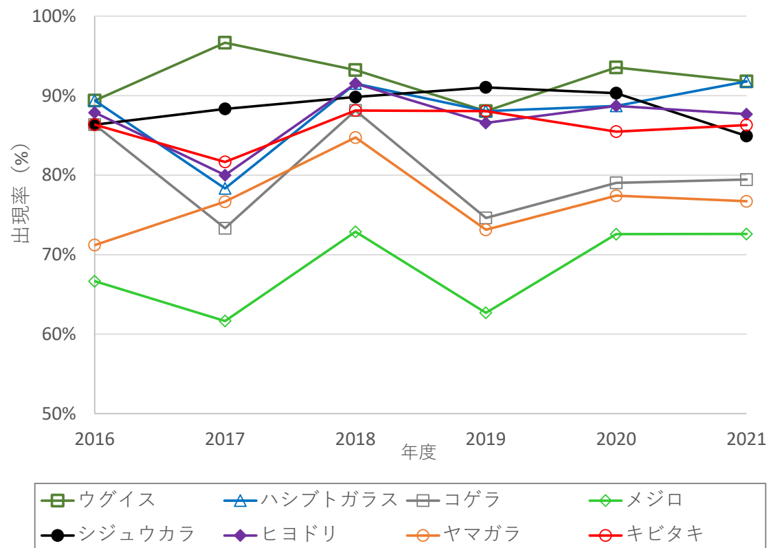
図Ⅲ-2-1. 出現率上位種における過去6年間（最新年度+過去5年）の推移（森林・繁殖期）
