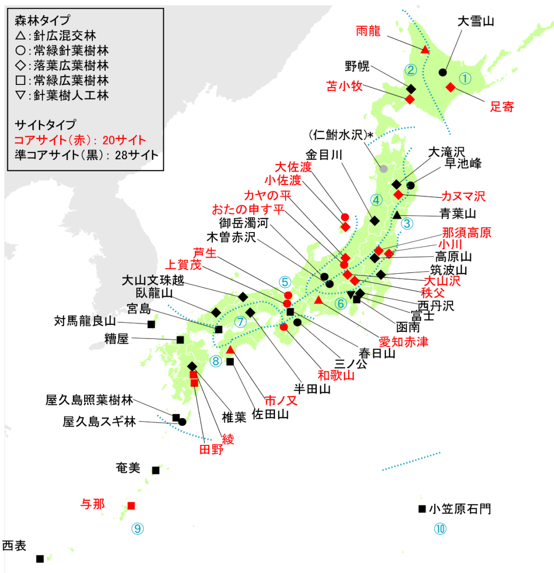
図Ⅱ-1-2. 第4期におけるモニタリングサイト1000森林・草原調査のコアサイト・準コアサイト
