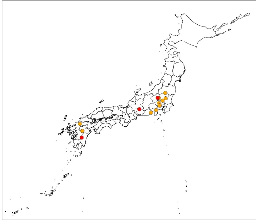
図Ⅲ-2-3. 繁殖期におけるガビチョウの確認サイト（●は、新規確認サイト）
