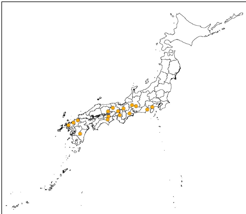
図Ⅲ-2-4. 繁殖期におけるソウシチョウの確認サイト
