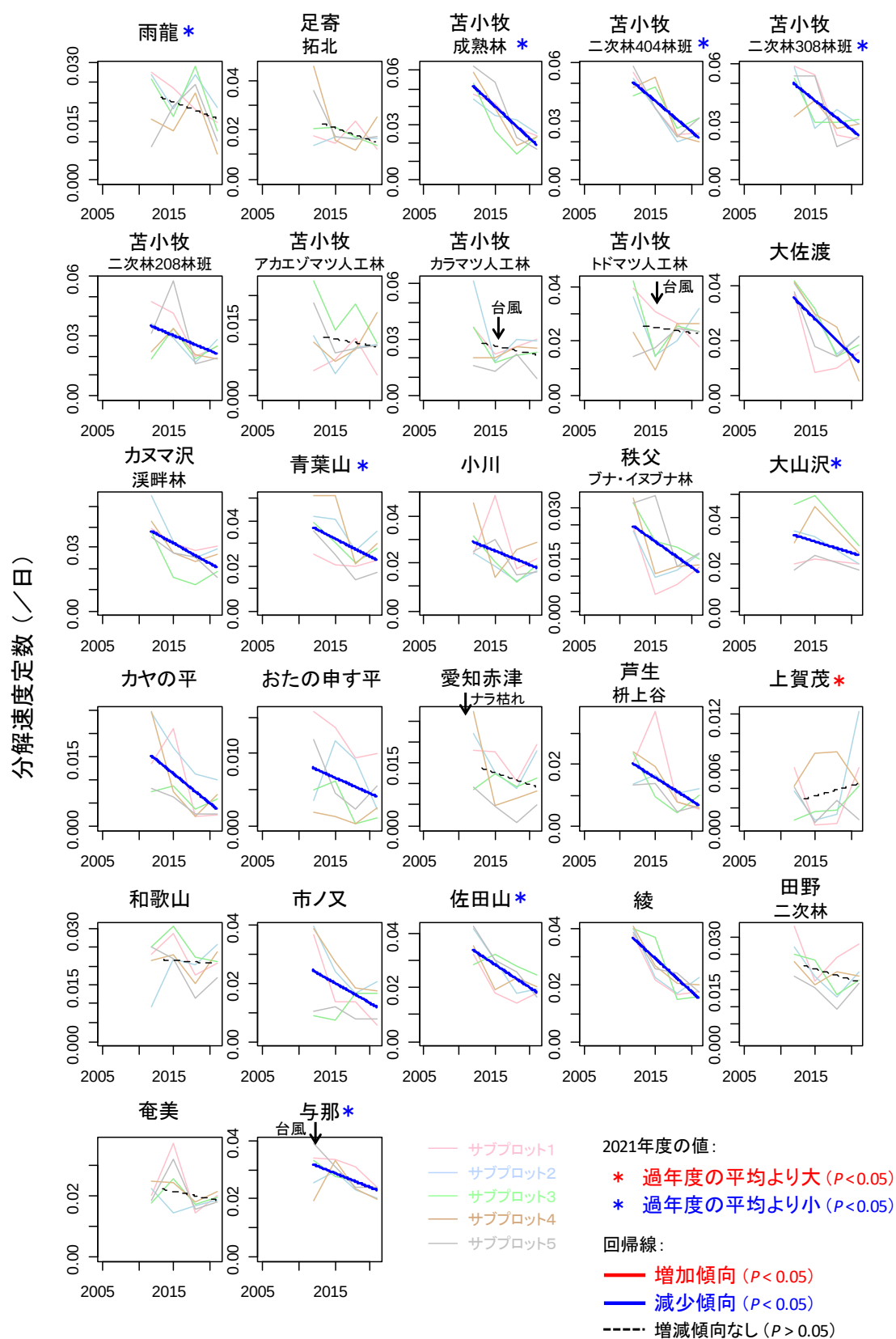
図Ⅱ-4-5. 各調査区における夏季のセルロース分解速度定数(堆積落葉層と土壌の平均値)の年変動
