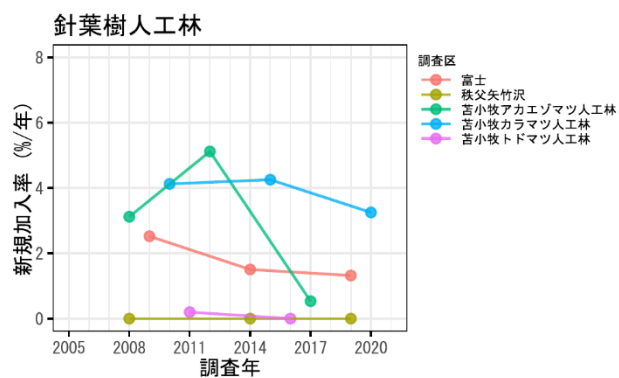
図Ⅱ-2-4. 各調査区における新規加入率の時系列変化
