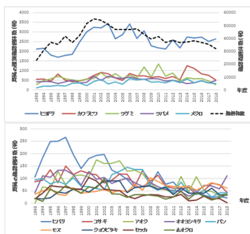
出典) 足立区, 2019: 令和元年度野鳥モニターによる足立区野鳥調査報告書より作成 図 II-17 足立区における鳥類の確認個体数の推移
