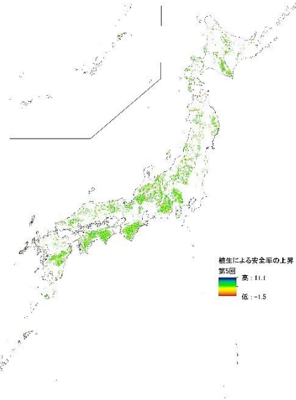
森林による安全率の上昇
