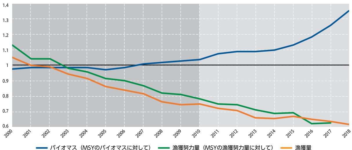
図6.3 正式な資源評価の対象となる漁業における相対的なバイオマス、漁獲努力量及び漁獲量の傾向 14
