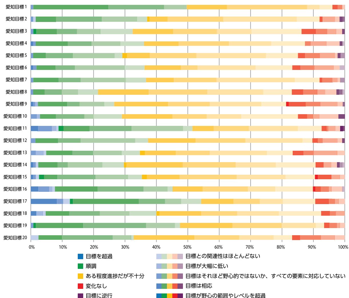
図21.2 国別目標に向けた進捗状況の評価と、これらと愛知目標の整合性
