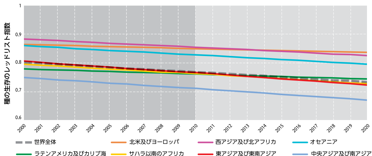
図12.1 世界全体及び地域レベルでのレッドリスト指数の傾向
