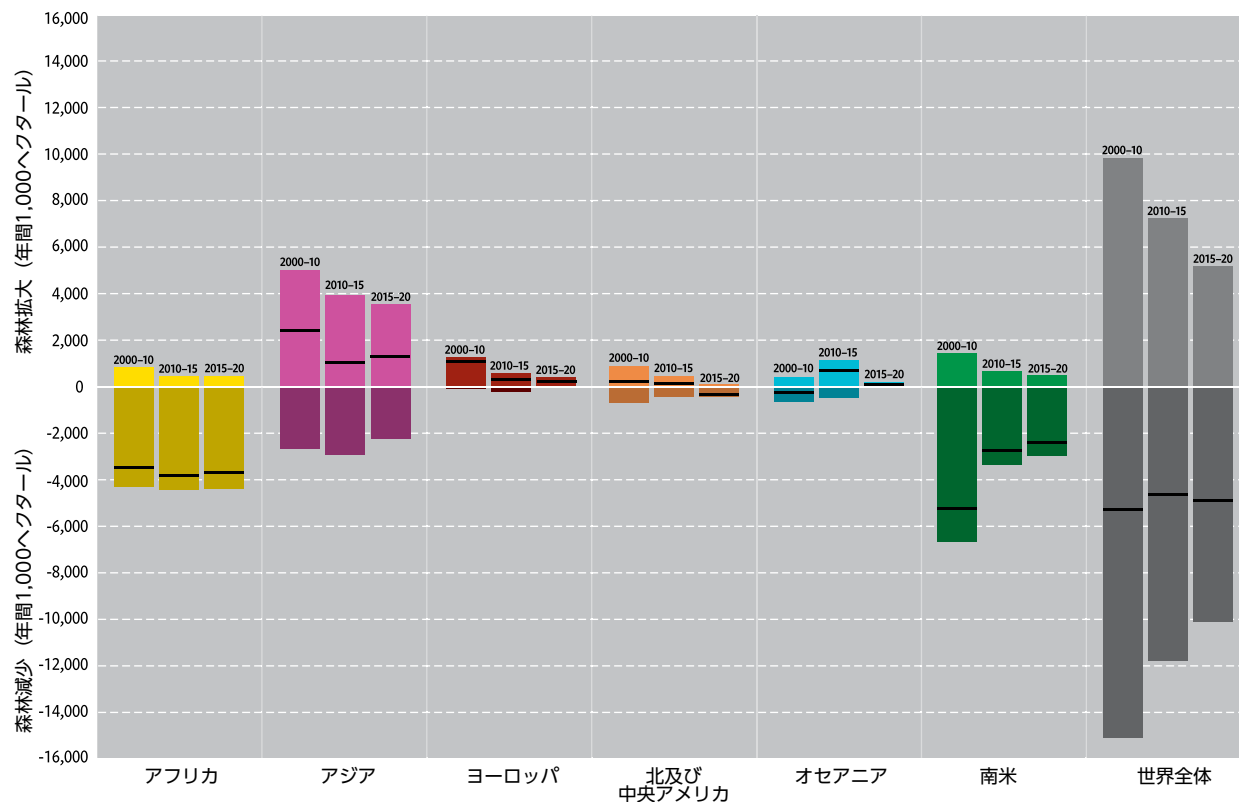
図5.1 世界の森林拡大と森林損失の年間速度 2
