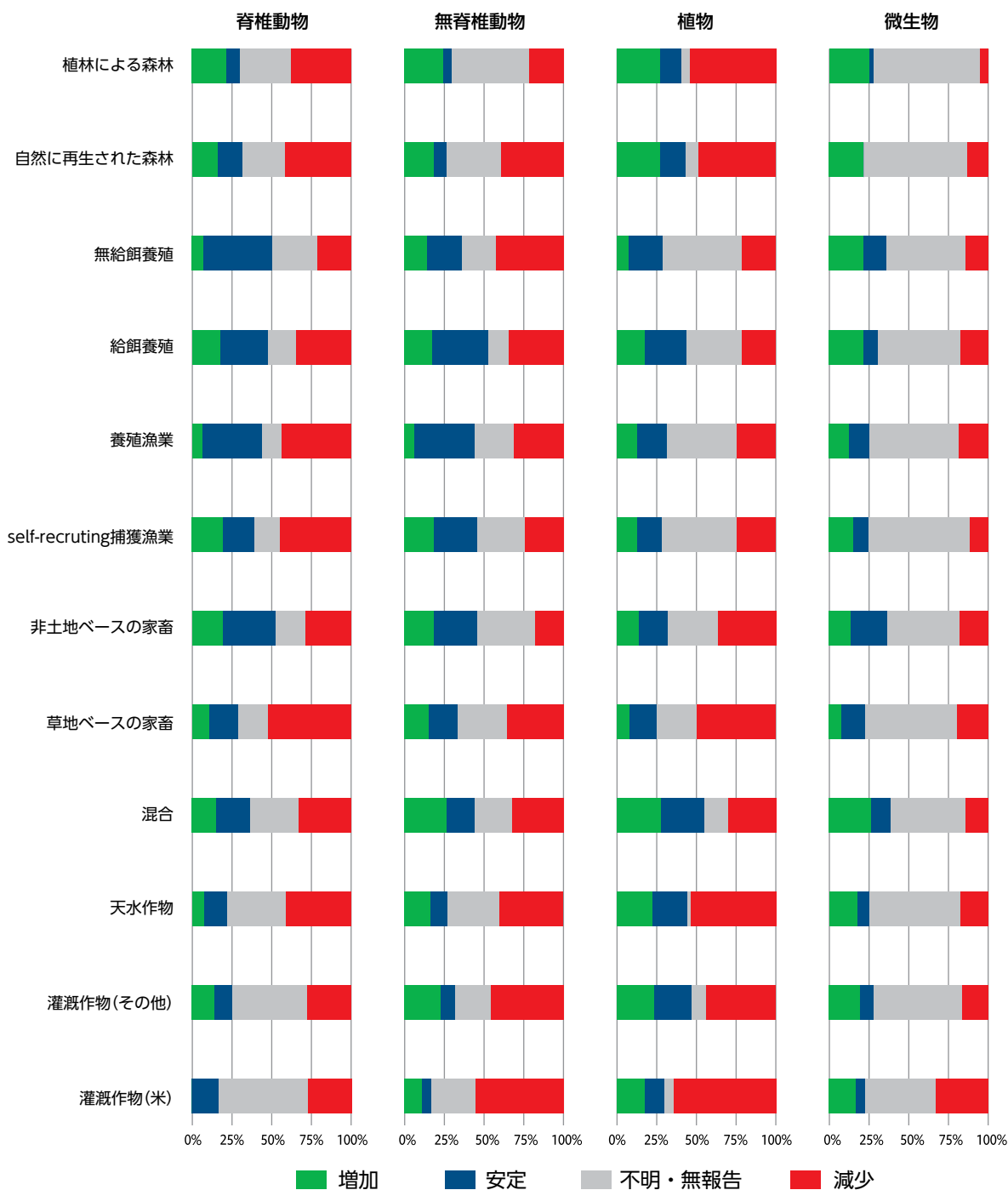
図7.2 食料・農業のための生物多様性白書（2019）のために作成された91か国の報告書に基づいた、さまざまな生産システムに関連する生物多様性の状況 22
