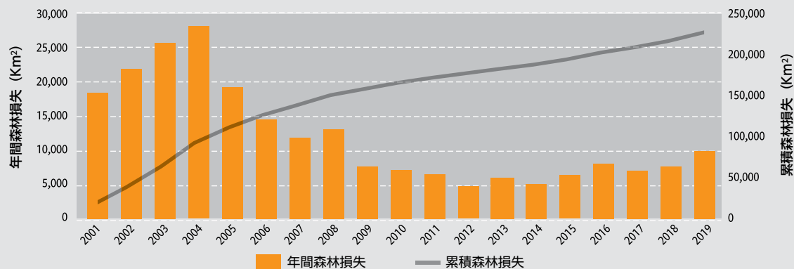
図5.3 ブラジルのアマゾンの年間森林減少面積 10
