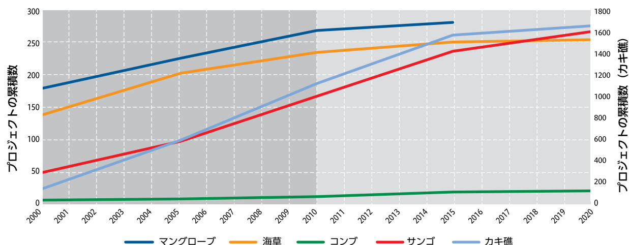
図15.1 2000年から2020年までに報告された海洋修復プロジェクトの累積数。カキ礁修復プロジェクトの数は、右軸のスケールによる。 28
