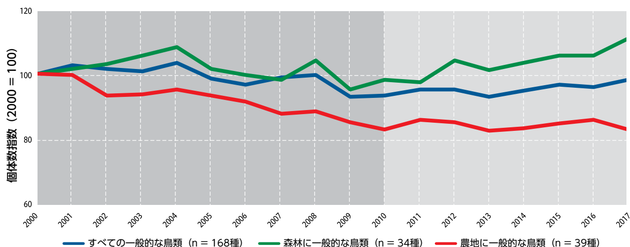
図7.1 ヨーロッパ野鳥指標
