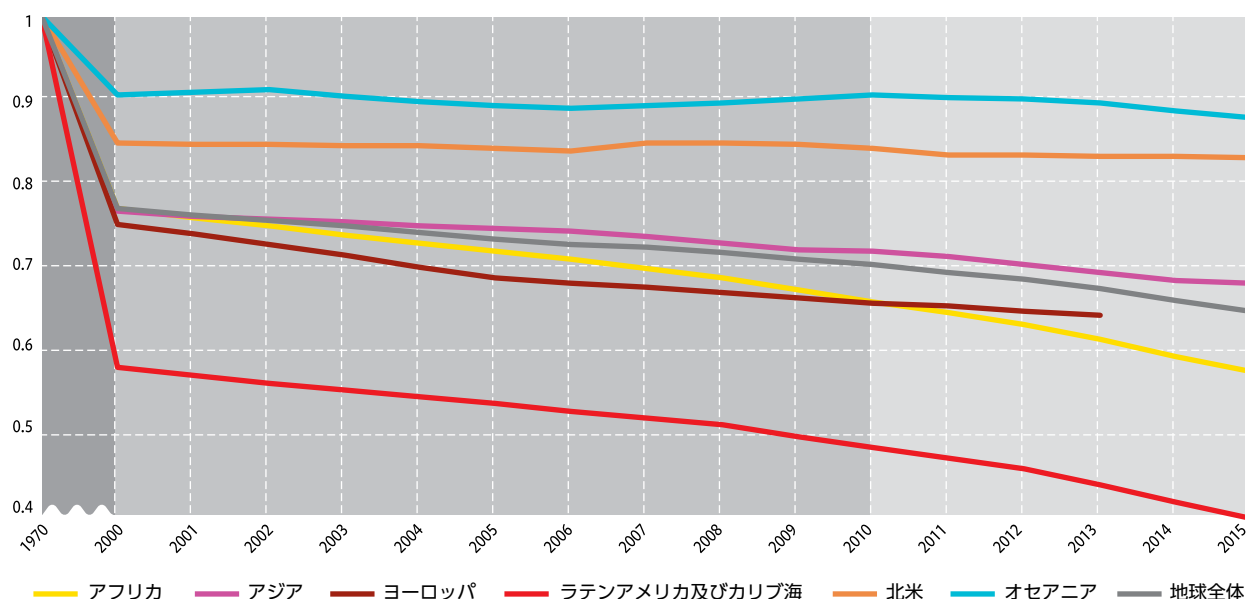
図5.4 1970年と比較した湿地範囲傾向（WET）指数は、6つの地域及び世界全体の自然湿地の範囲について、2000年から2015年までの変化を示している。 4
