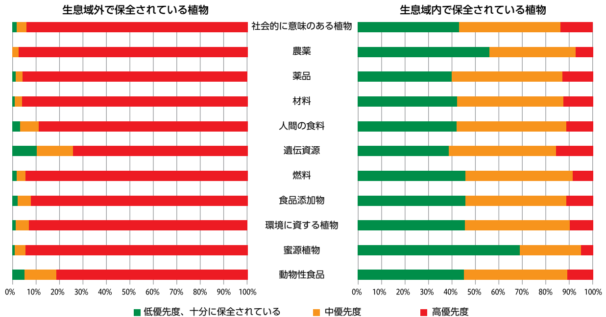
図13.1 野生植物の保全状況
