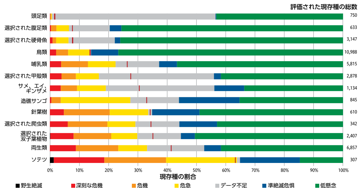
図12.2 さまざまな分類学的グループにわたるIUCNレッドリストのさまざまな絶滅危惧カテゴリの種の割合
