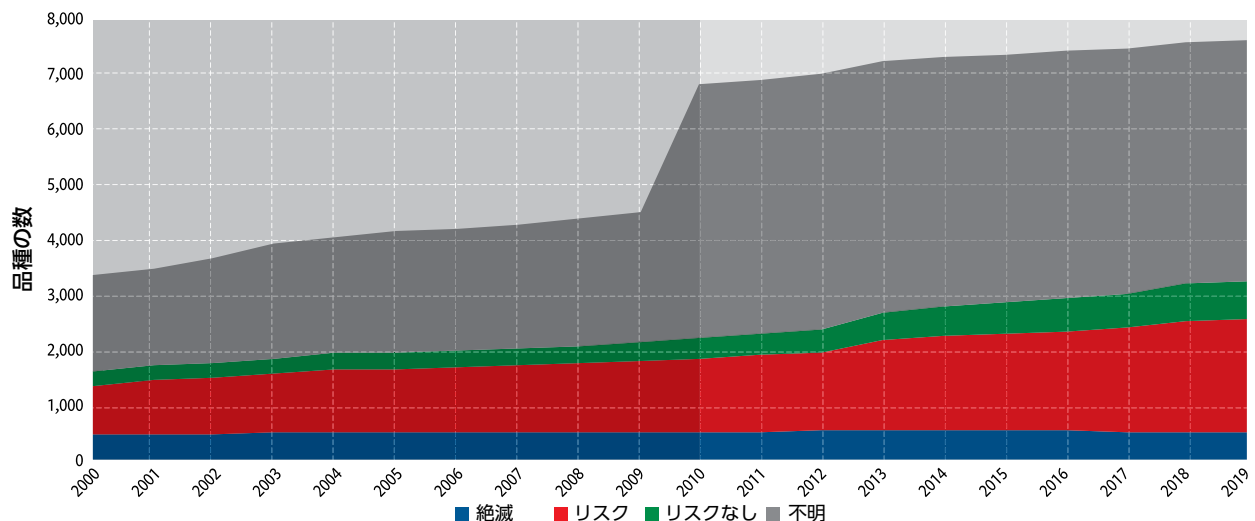
図13.2 リスクカテゴリー別ローカル品種の状況の傾向
