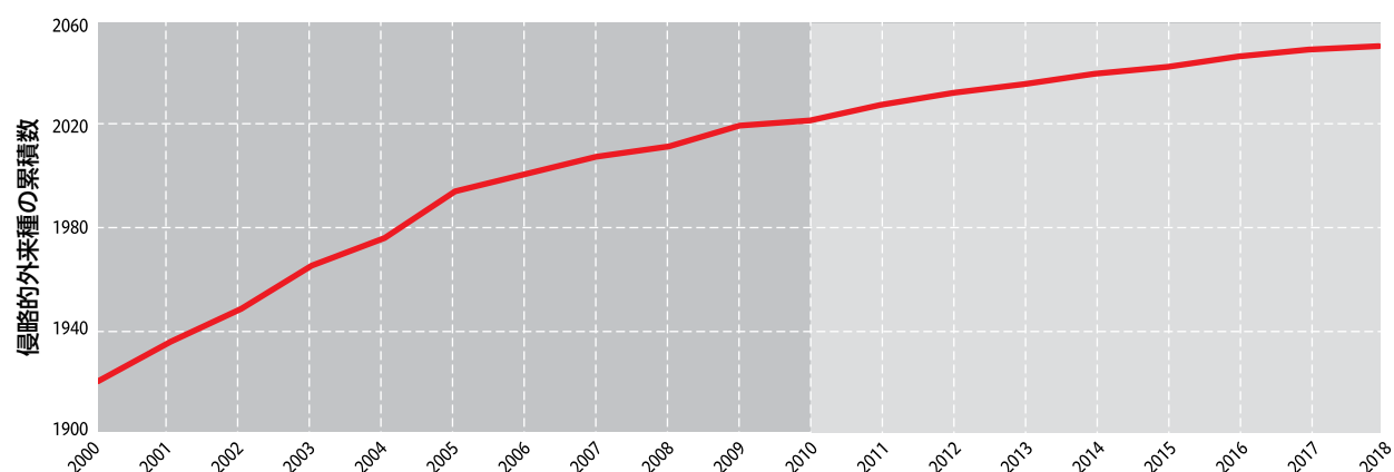
図9.2 侵略的外来種の累積数の世界的傾向
