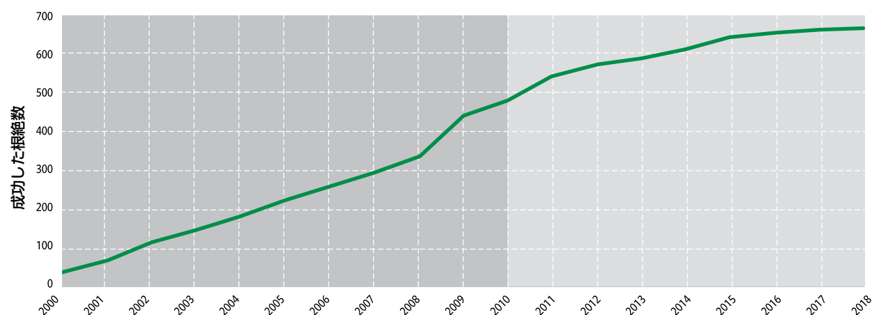
図9.1 全島嶼で2000年以降の年ごとに成功した外来哺乳類根絶プロジェクトの累積数 6
