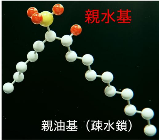
バイオIOS 分子構造モデル
