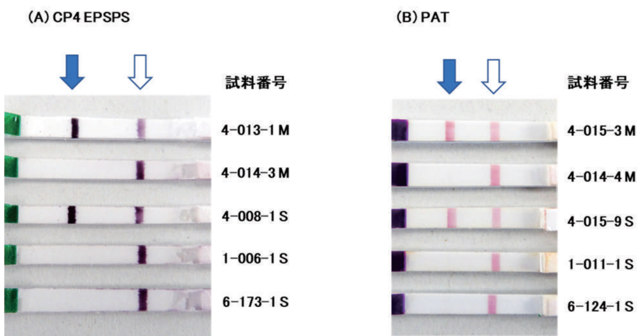
図 2 免疫クロマトグラフ法によるグリホサート耐性タンパク質CP4 EPSPS(A) 及びグルホシネート耐性タンパク質PAT(B)の検出の例
