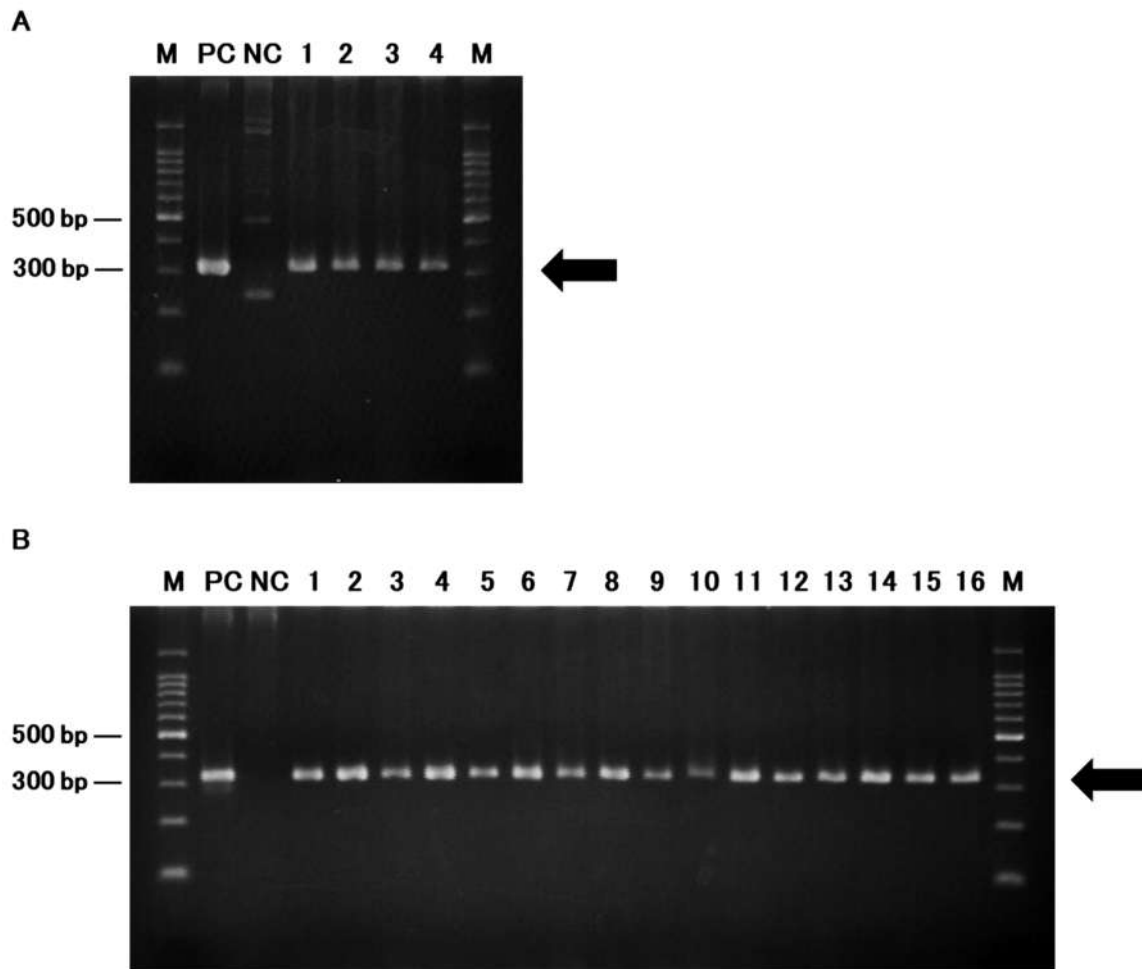
図 3 PCR による cp4 epsps 遺伝子(A)および bar 遺伝子(B)の検出結果
