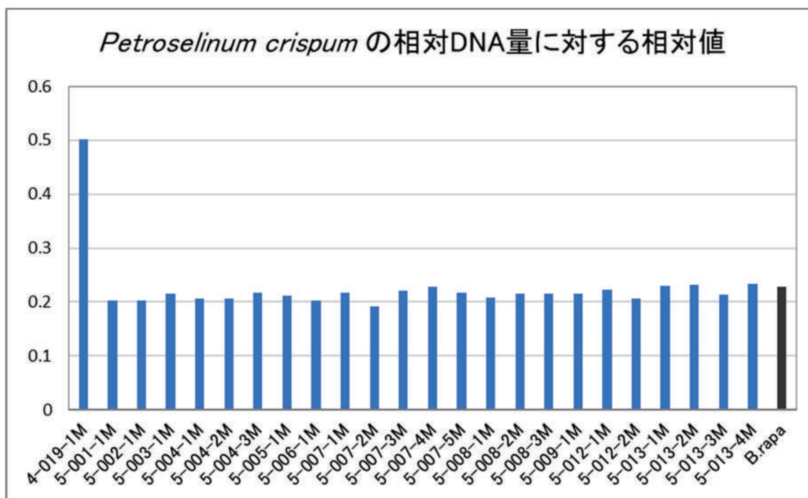
図 1 母植物葉を用いた FCM 解析
