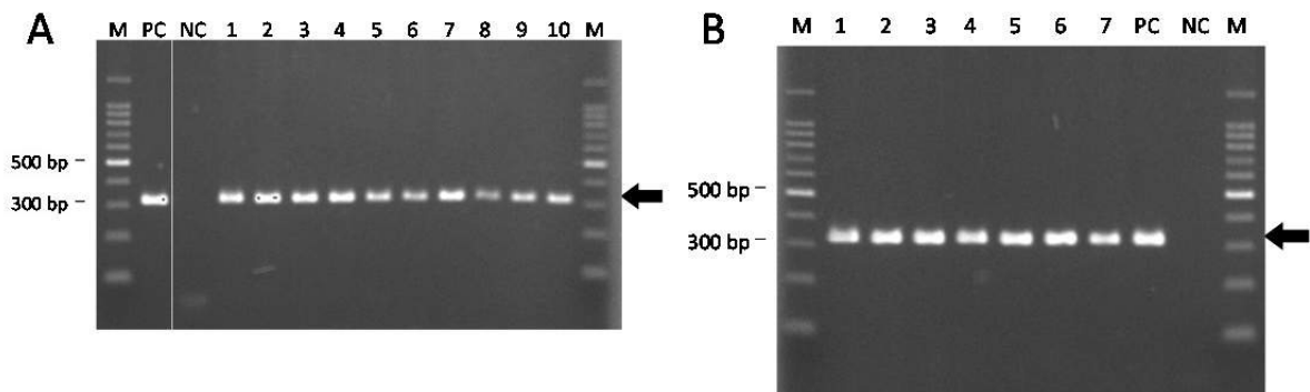
図 1-3 PCR による cp4 epsps 遺伝子(A)及び bar 遺伝子(B)の検出の例
