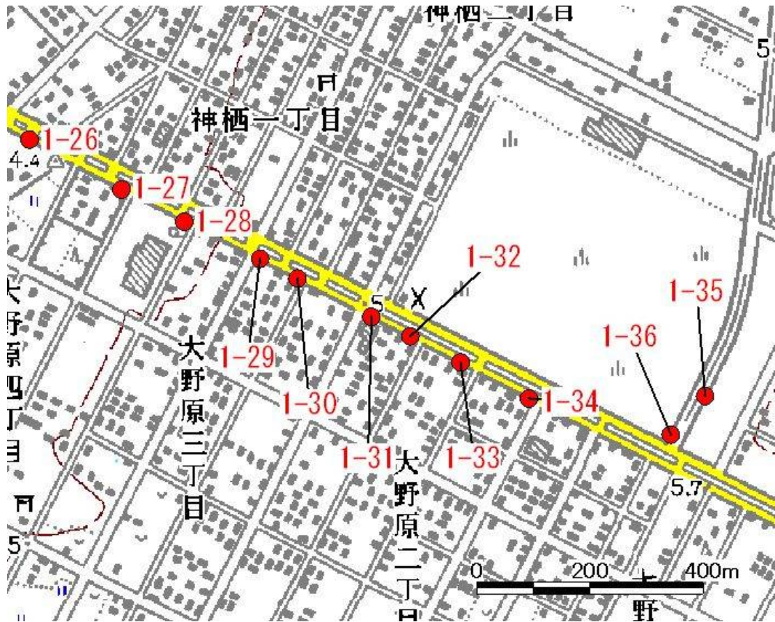
図3 神栖市平泉交差点～木崎西交差点付近の採取地点と遺伝子組換え体の分布
