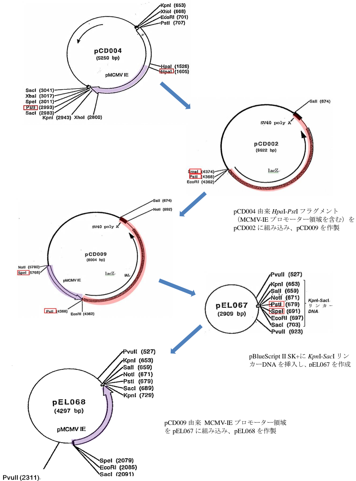
図6 プラスミド pEL068 の作製
