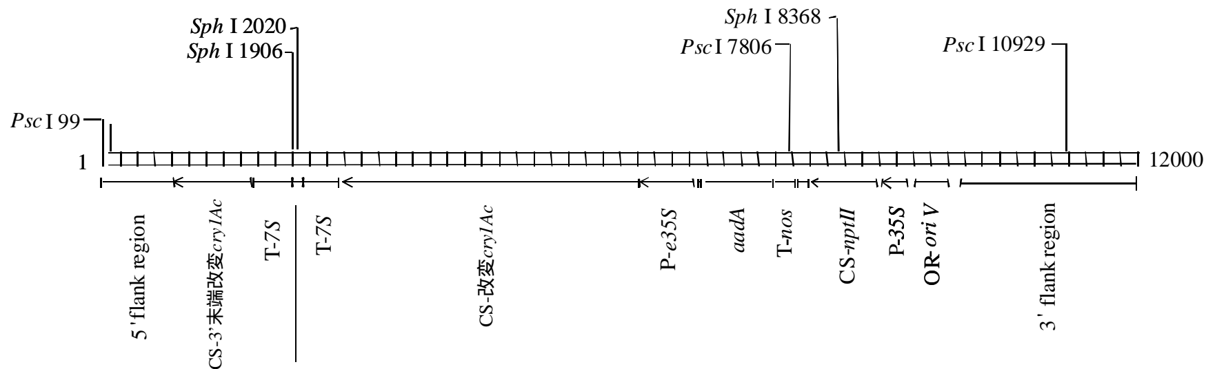
図 3 15985 の育成に用いられた 531 の導入遺伝子地図 7
