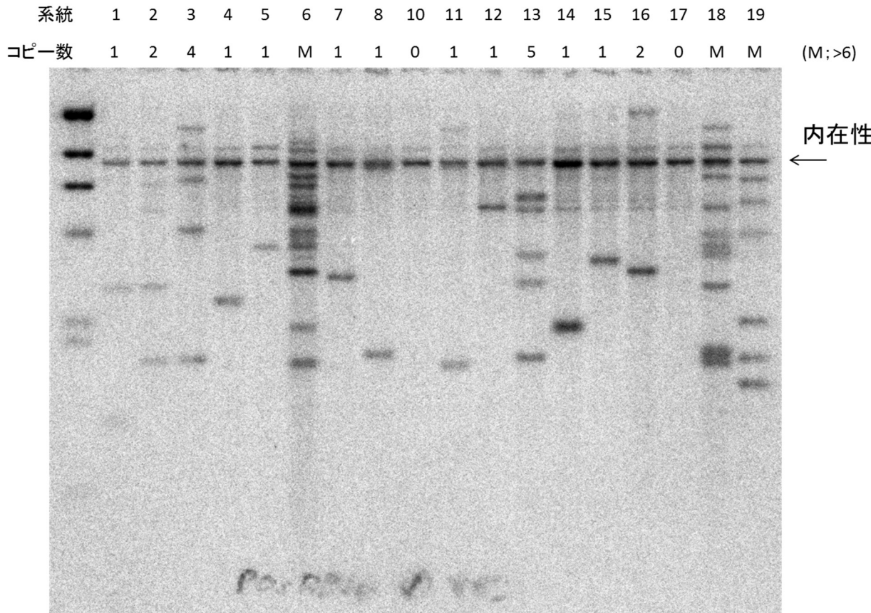
図2 移入核酸の検出 T 0 世代。HindIII消化。プローブ：WRKY45断片。
