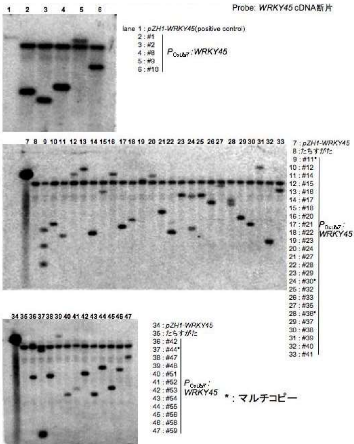
図2 移入核酸の検出 T 1 世代。HindIII 消化。プローブ: WRKY45 断片
