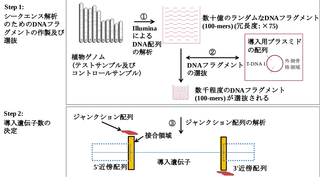
図 12 NGS/JSA の解析手法の概念図 (Kovalic et al., 2012) 71
