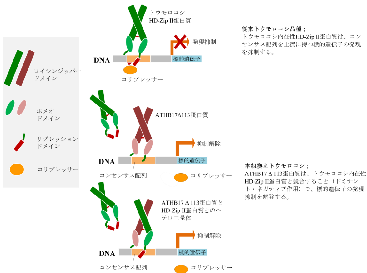
図 5 ATHB17 \Delta 113 蛋白質のドミナント・ネガティブ作用によって生じると考えられる、HD-Zip II 蛋白質による標的遺伝子の発現抑制の解除を示した模式図 26 プロモーター領域にコンセンサス配列をもつトウモロコシ内在遺伝子が複数存在することが、本組換えトウモロコシを供試した RNA シークエンス解析及びその結果を基におこなったバイオインフォマティクス解析によって明らかになっている。詳細は、第一の 2-(1)-ロ-②-3-2)-(B) (p45) に記載した。
