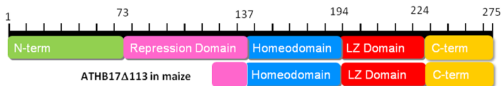
図 4 シロイヌナズナにおいて発現する完全長の ATHB17 タンパク質 (上段) 及び本組換えトウモロコシにおいて発現する ATHB17Δ113 タンパク質 (下段) の模式図 24
