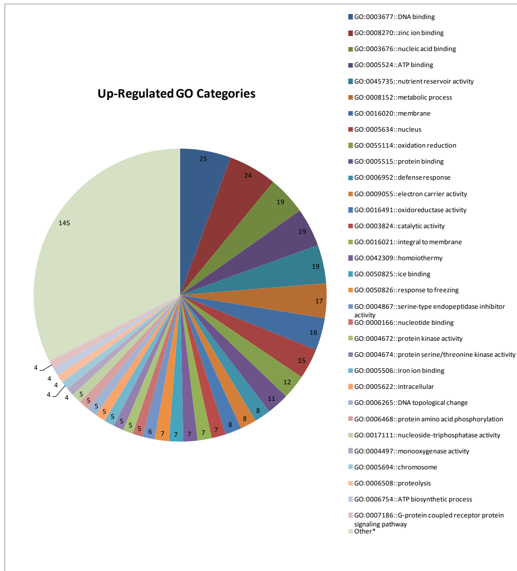
図 8 RNA シークエンス解析において発現が増加していた転写産物の GO カテゴリ — 39
