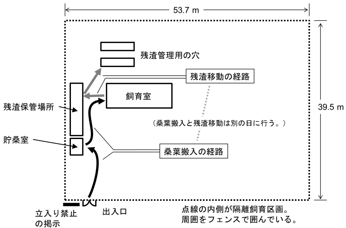
図3. 隔離飼育区画内の施設の概要
