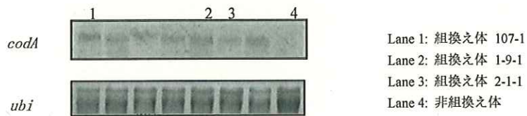
図 1 codA 遺伝子の発現
