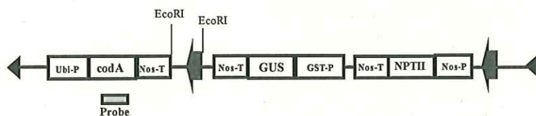
図 1 サザンハイブリダイゼーション
