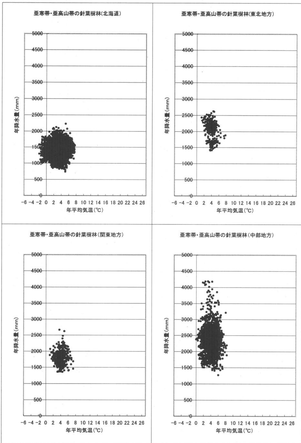
図Ⅱ.5.5 亜寒帯・亜高山帯の針葉樹林（自然植生）と環境要因(気温、降水量)との関係
