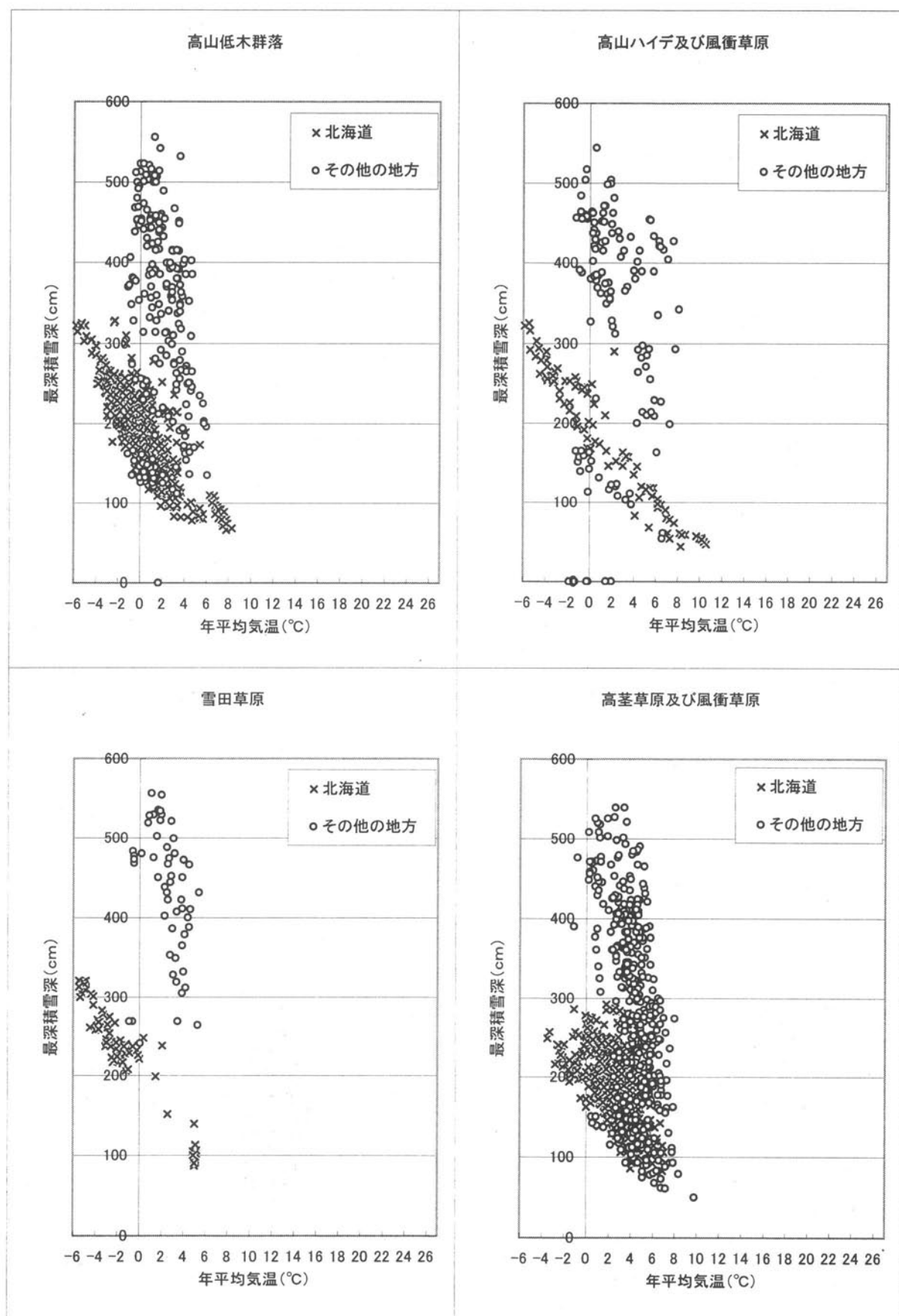
図II.5.2 寒帯・高山帯・亜寒帯・亜高山帯の主な自然植生と環境要因(気温、最深積雪深)との関係
