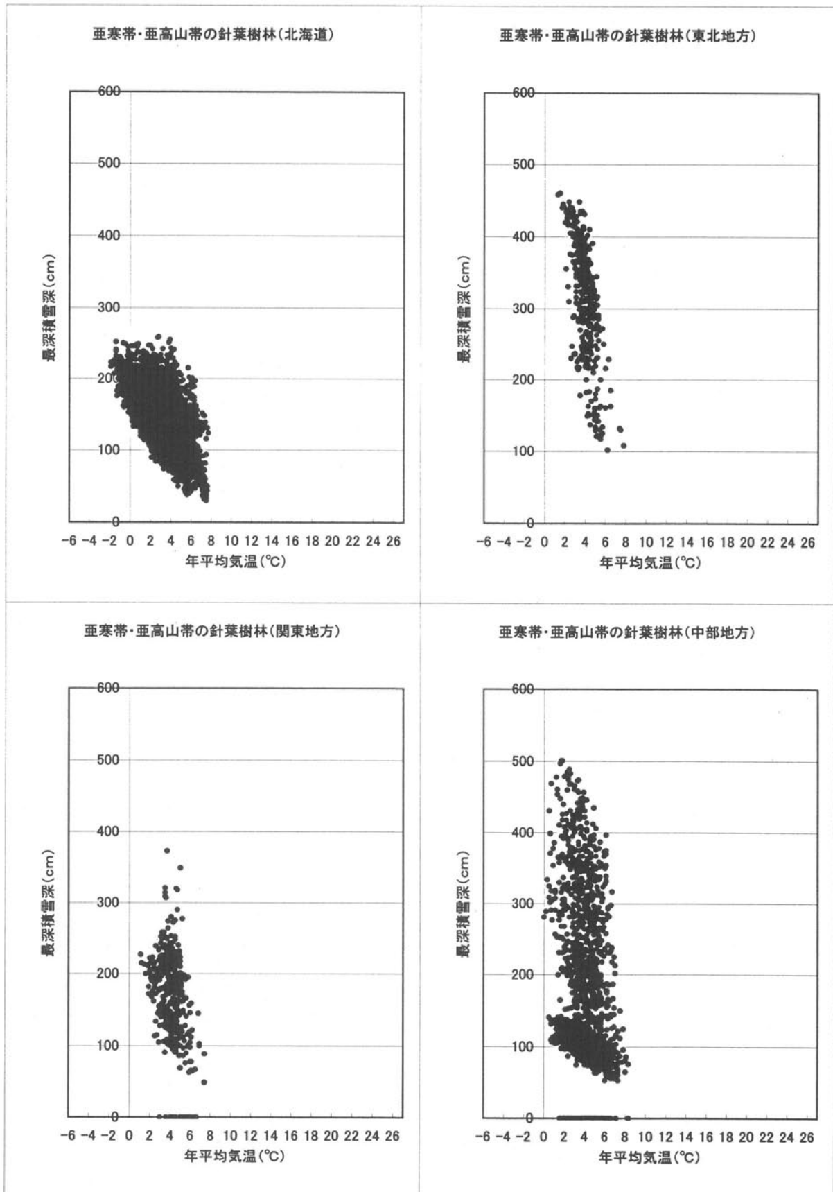
図Ⅱ.5.6 亜寒帯・亜高山帯の針葉樹林（自然植生）と環境要因(気温、最深積雪深)との関係
