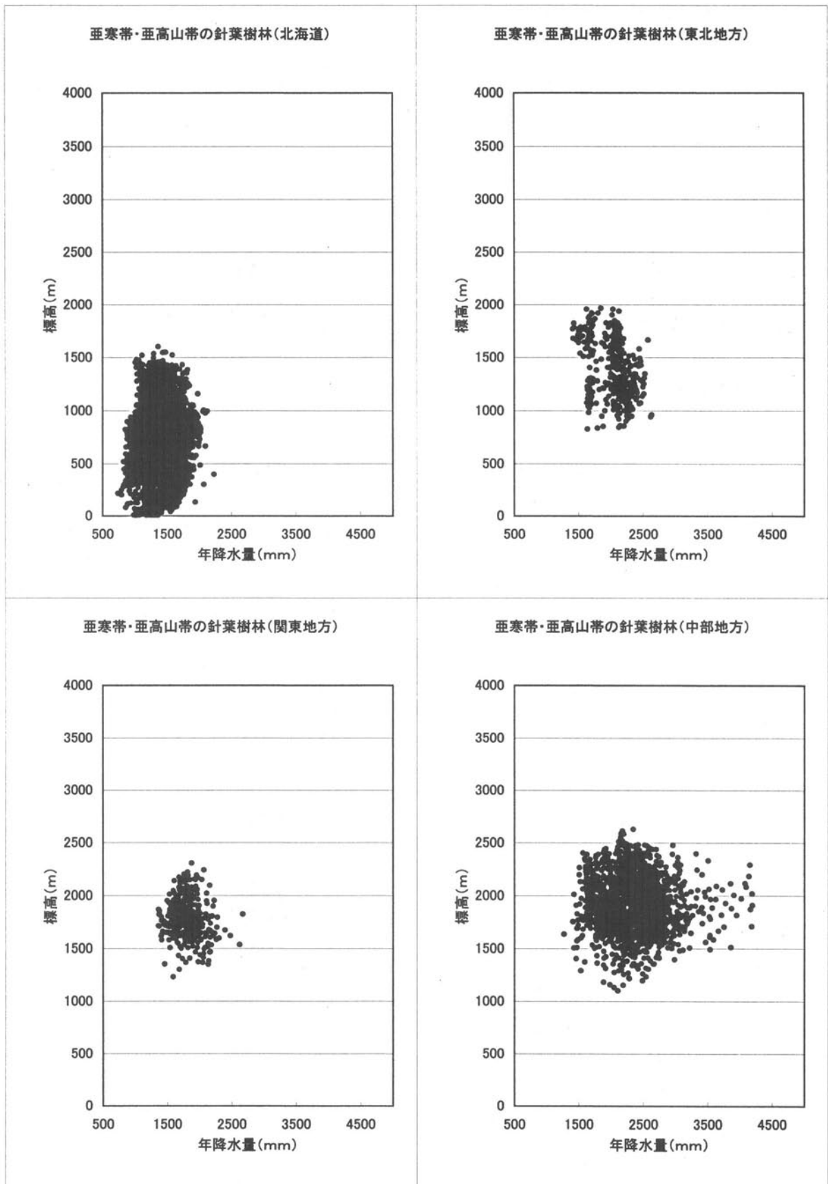
図Ⅱ.5.8 亜寒帯・亜高山帯の針葉樹林（自然植生）と環境要因(降水量、標高)との関係
