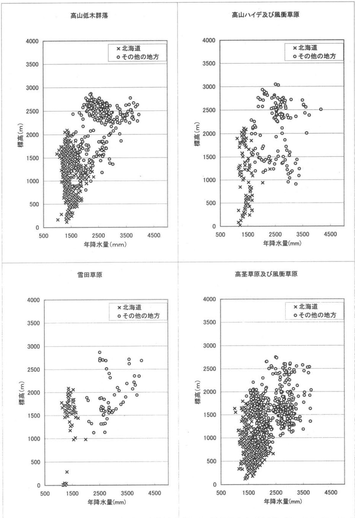
図Ⅱ.5.4 寒帯・高山帯・亜寒帯・亜高山帯の主な自然植生と環境要因(降水量、標高)との関係
