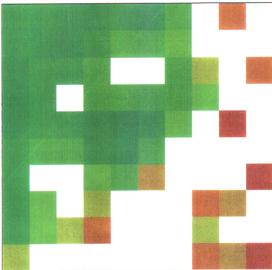
図1-11-1 対象地域のCON値分布図
