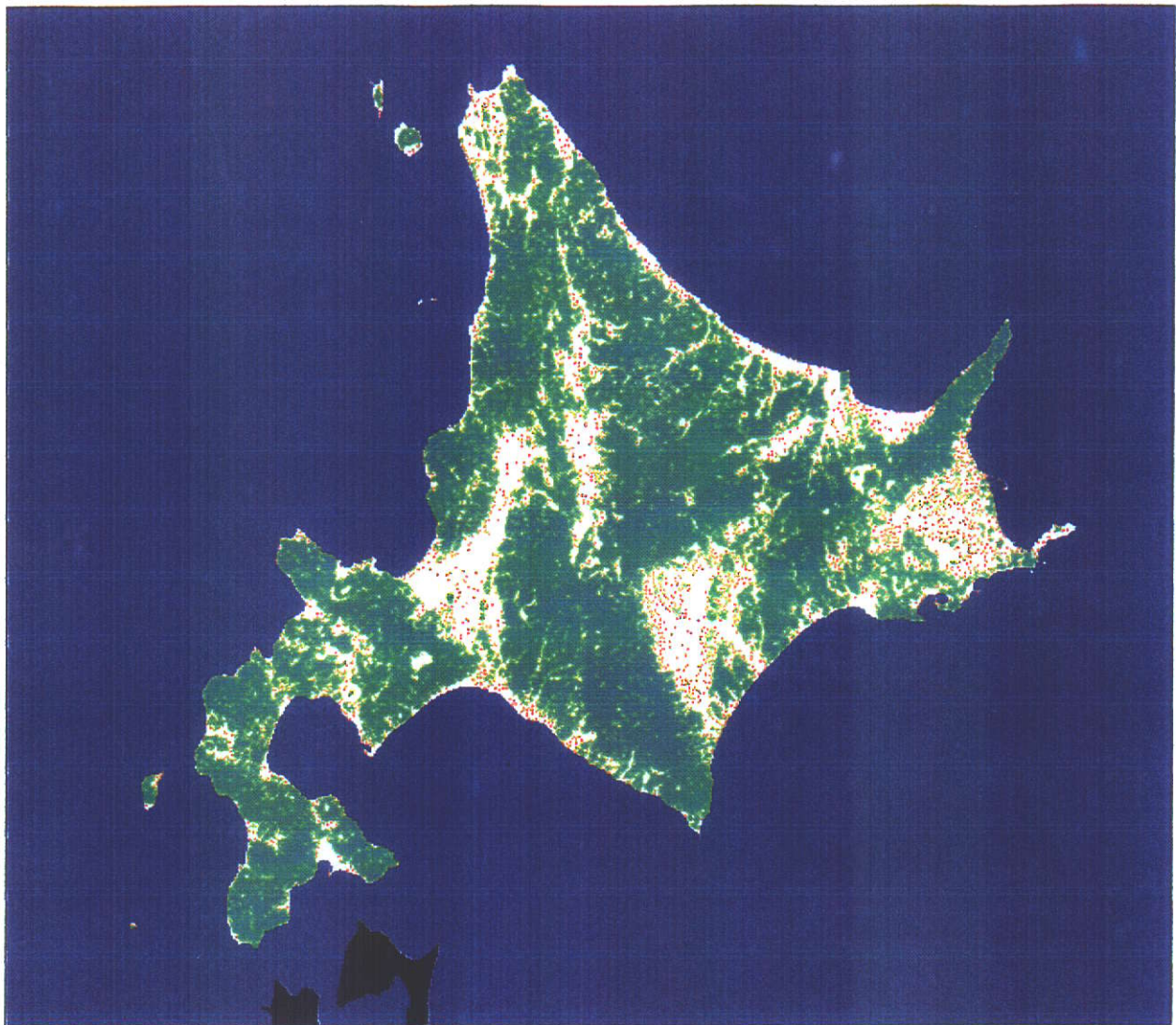
図1-11-4 北海道地方のCON値分布図
