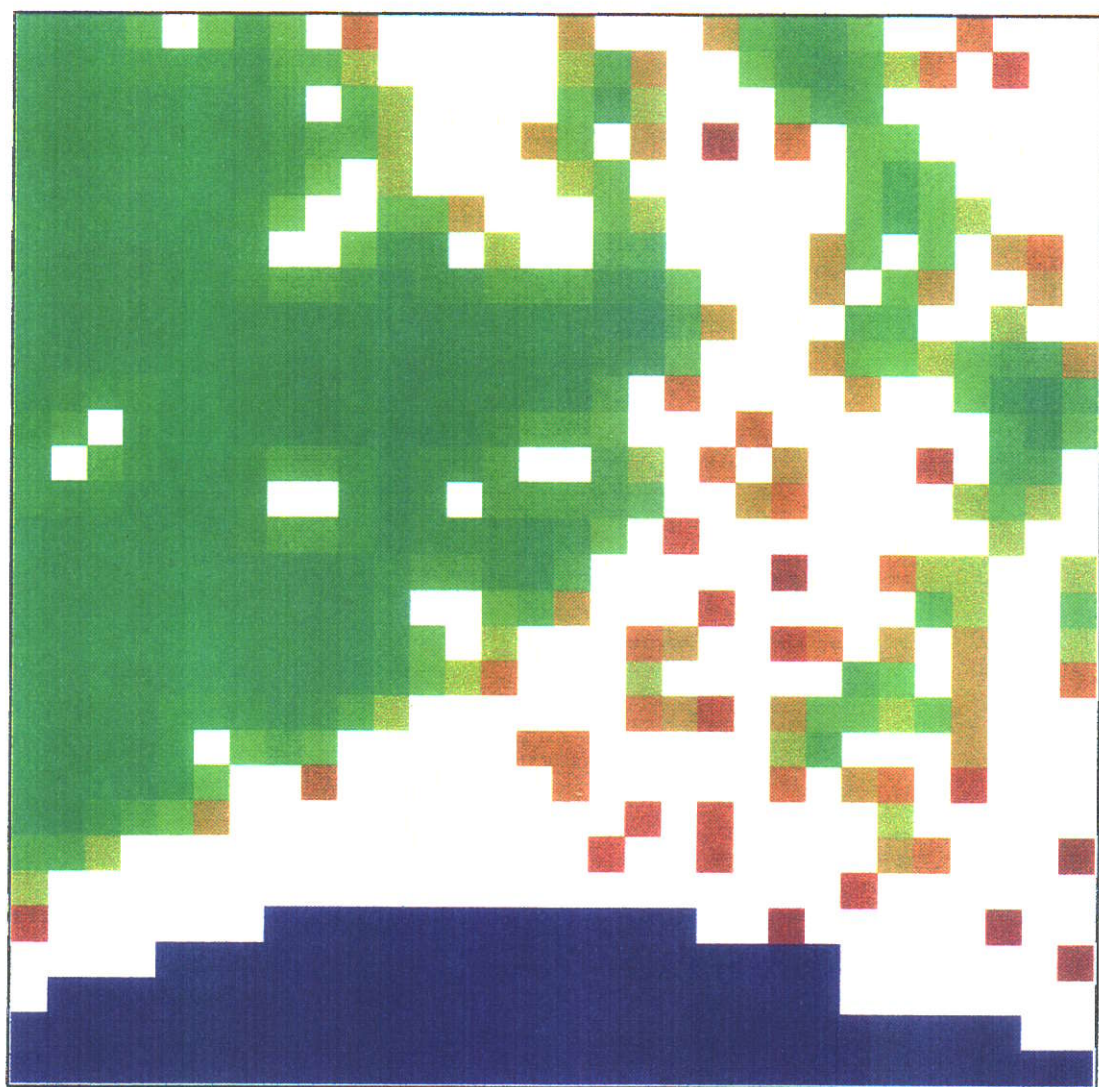
図1-11-2 対象地域周辺10km×10km範囲のCON値分布図
