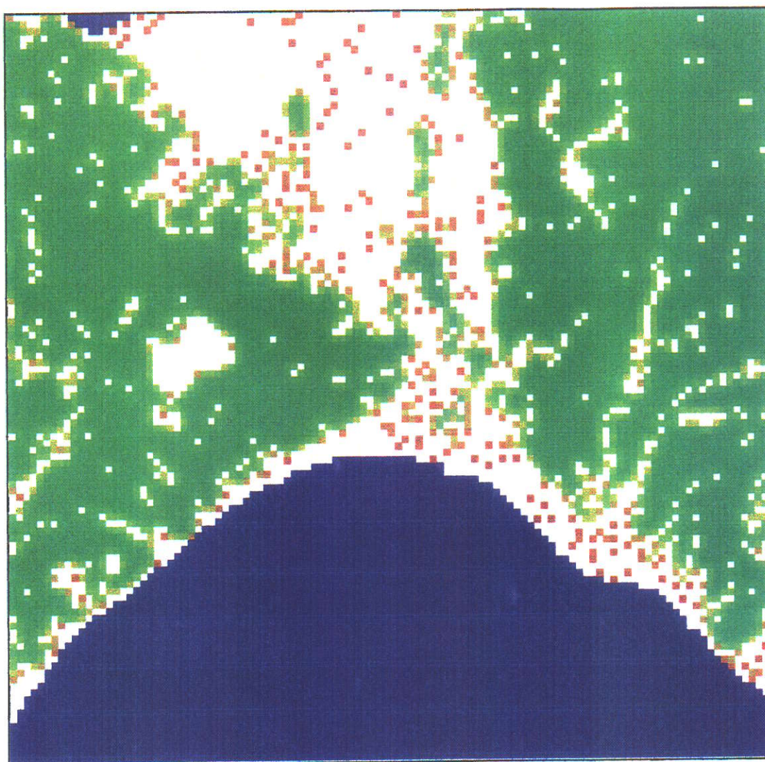
図1-11-3 対象地域周辺50km×50km範囲のCON値分布図
