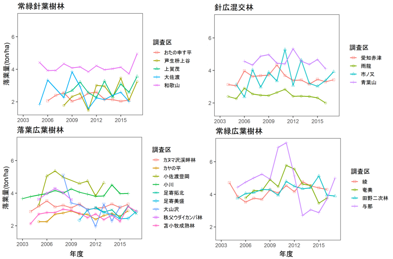
図 II-1-3. 森林タイプ毎の年間落葉量の年変動
