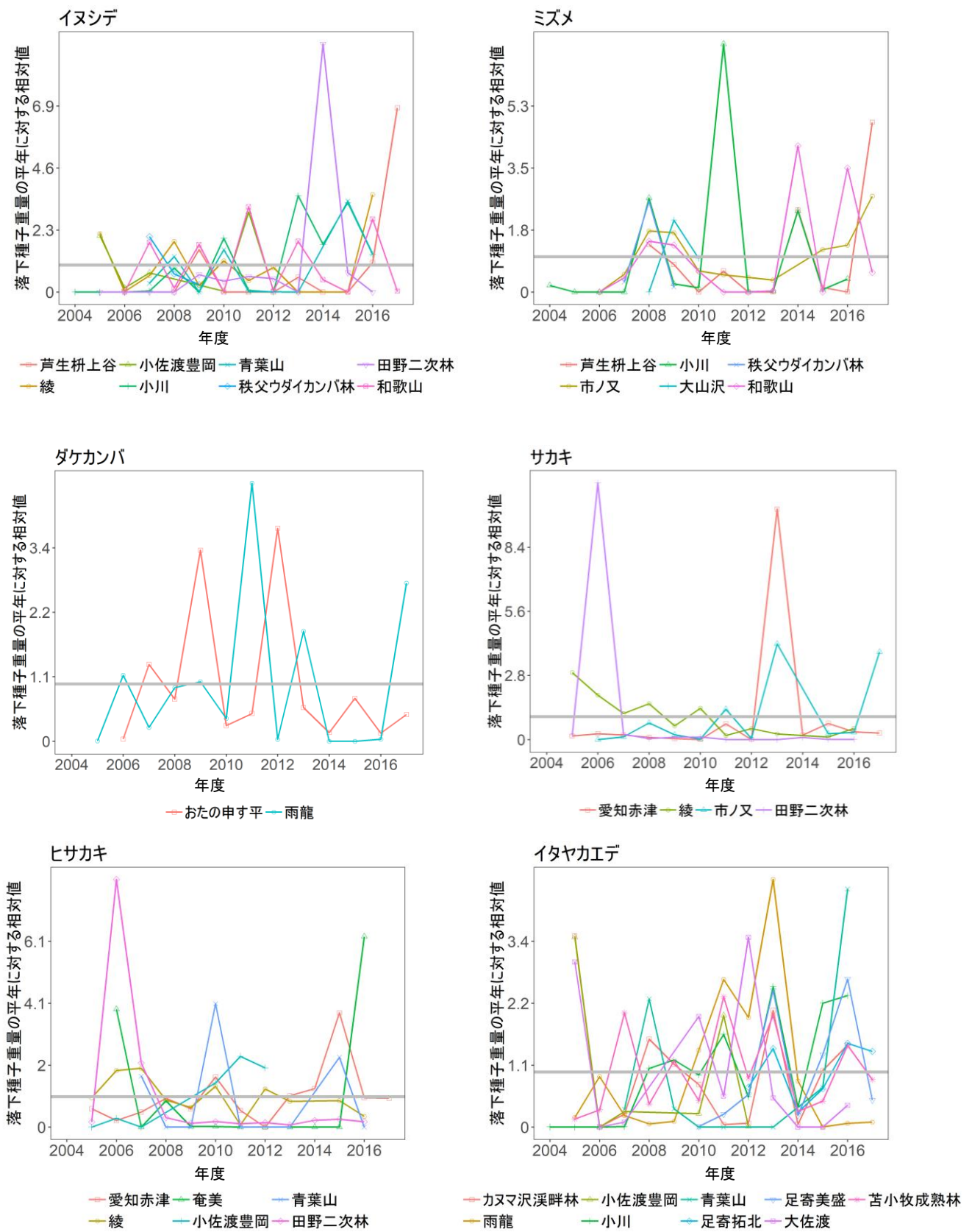
図II-1-4. 主要樹種の2004～2017年の各年度の落下種子重量(続き)
