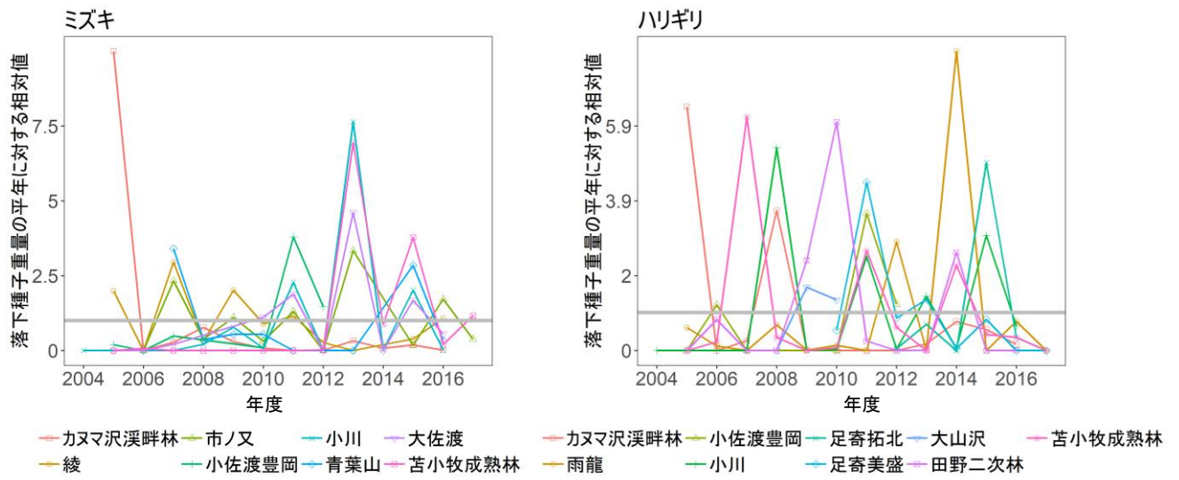
図II-1-4. 主要樹種の2004～2017年度の各年の落下種子重量(続き)
