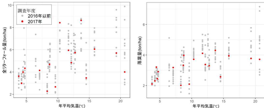
図 II-1-1. 2004～2016 年度(灰色)及び2017 年度(赤色)のリターフォール量及び年間落葉量と年平均気温の関係
