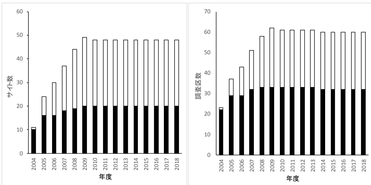
図 I-3-1. 2004-2018 年度のコアサイト・準コアサイト数及び調査区数の推移
