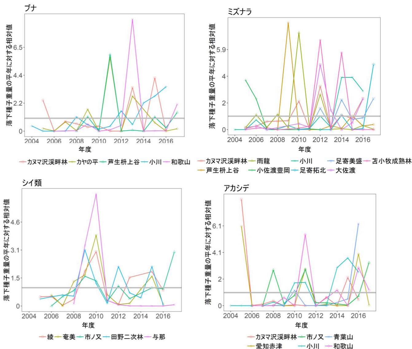
図II-1-4. 主要樹種の2004～2017年の各年の落下種子重量
