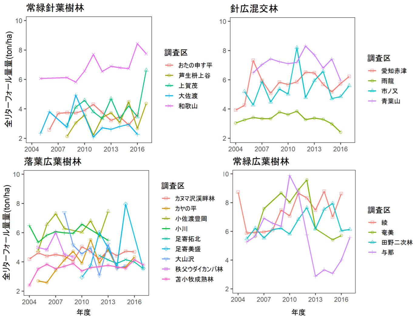
図 II-1-2. 森林タイプ毎の年間リターフォールの年変動
