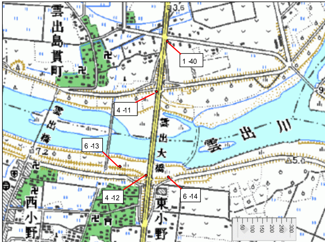
図 10 津市雲出大橋付近の採集地点 (1 / 2.5 万図 松阪港)
