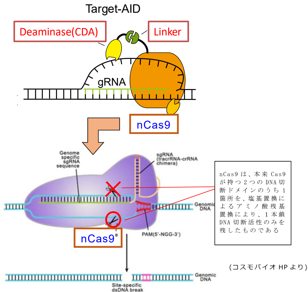
図 1 Target-AIDシステムによる標的遺伝子の塩基変換に必要なパーツ
