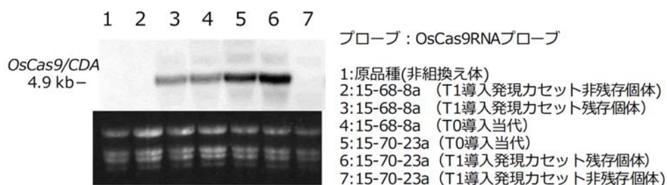
図5 ノーザンブロット解析による、個体間及び世代間での転写レベルにおける発現の有無(当該遺伝子組換え体T 0 世代は5レーン目)。
