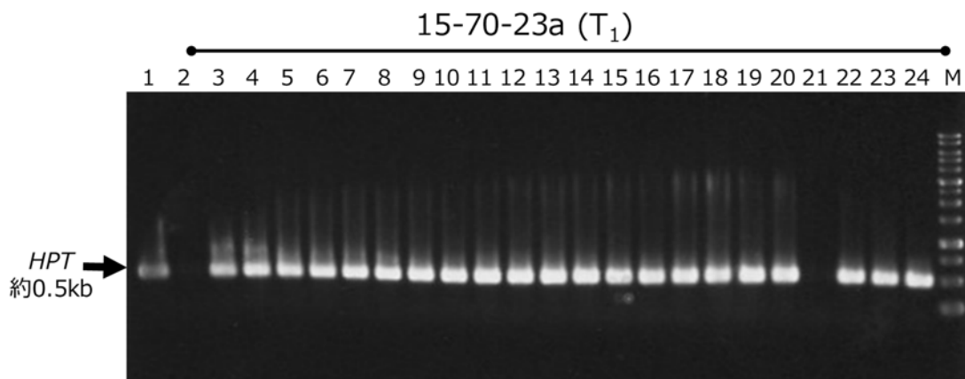
図3 先行系統(15-70-23a)のT 1 世代の種子24粒から発芽した個体における、HPT遺伝子の移入の有無。矢印の位置のバンドがPCR法で増幅した導入遺伝子であり、No.2及び21はHPT遺伝子を持たない。
