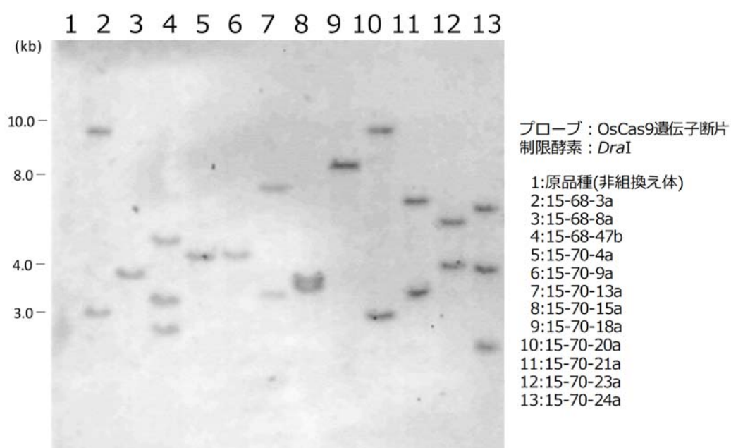
図4 サザンブロット解析を用いた移入核酸の検出による、移入コピー数の推定（全てT 0 世代、当該遺伝子組換え体は12レーン目）。
