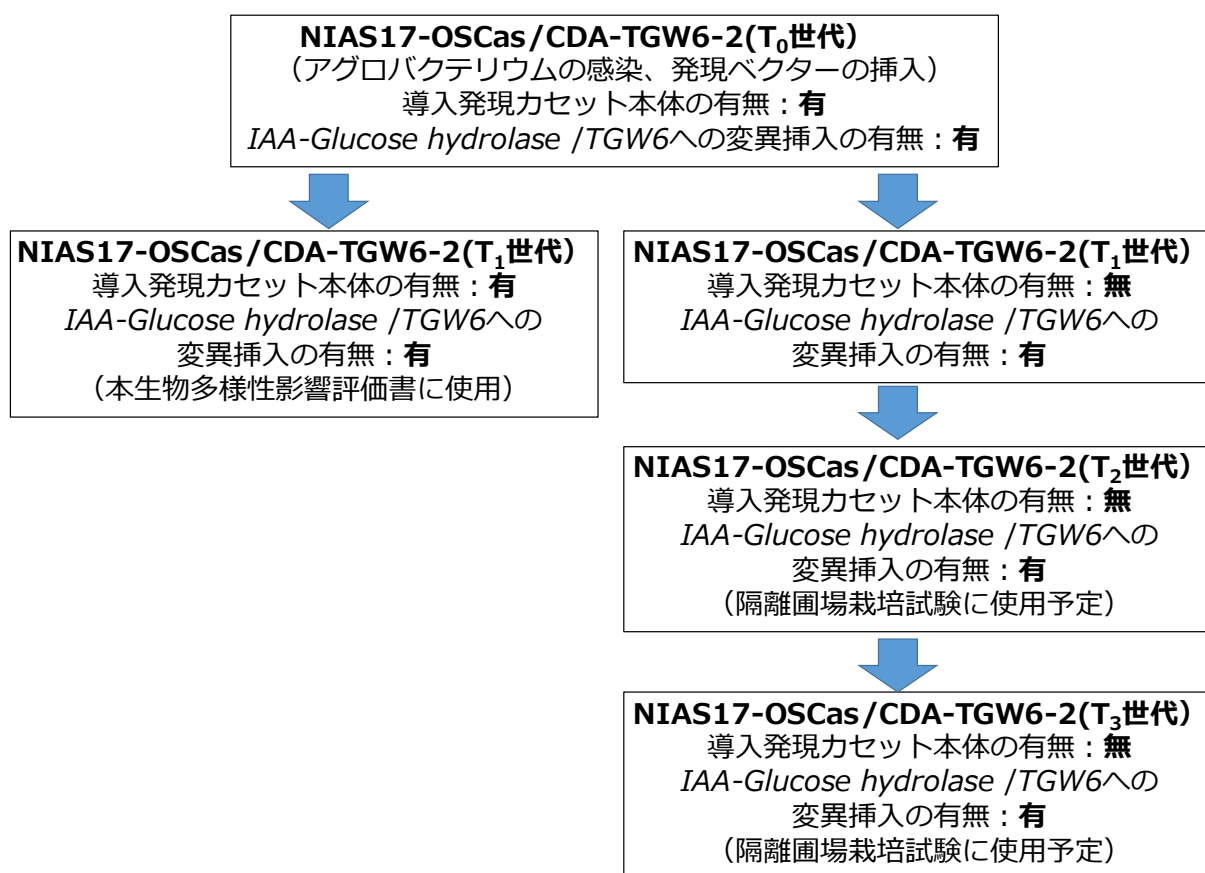
図 6、NIAS17-0SCas/CDA-TGW6-2 の系譜図
